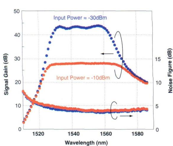
Рисунок А.3 – Зависимость коэффициента усиления и коэффициента шума от длины волны для усилителя диапазона С.
