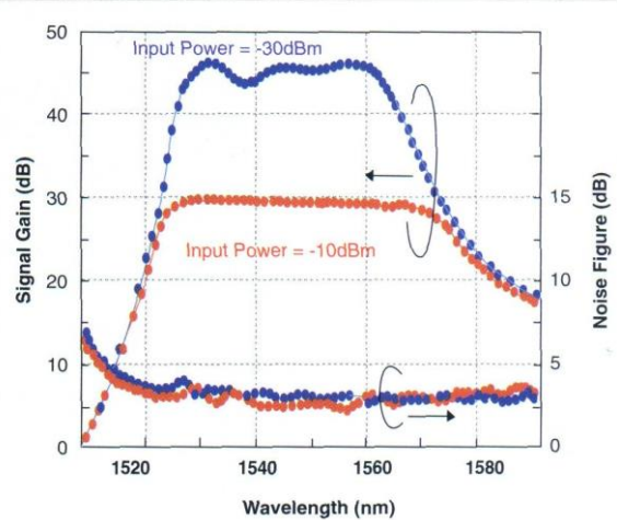
Рисунок А.4 – Зависимость коэффициента усиления и коэффициента шума от
