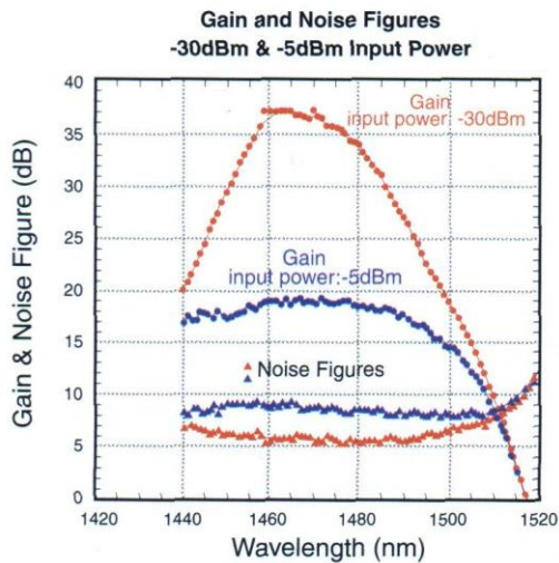
Рисунок А.2 – Зависимость коэффициента усиления и коэффициента шума для усилителя диапазона S от длины волны (рис. а, б) и от входной мощности сигнала (рис. в).
