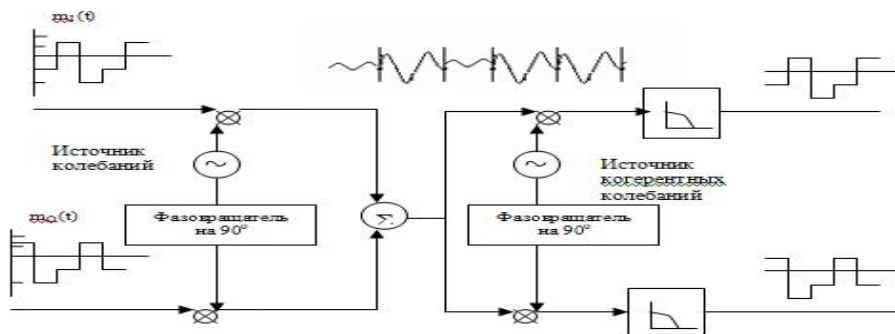
Рис. 1.72. Схема модулятора-демодулятора QAM
