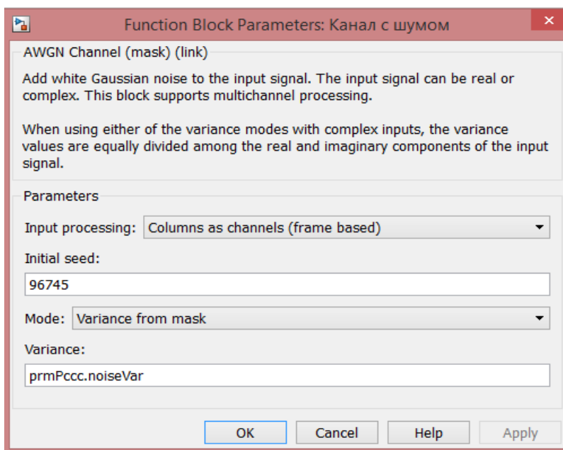
Рис. 3.151. Параметры блока «AWGN»
