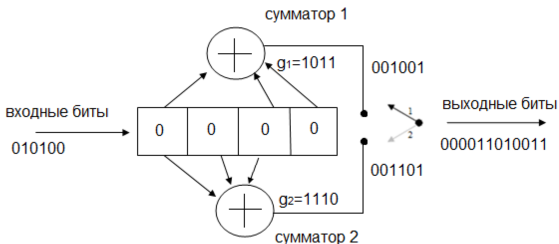
Рис. 3.85. Сверточный кодер
