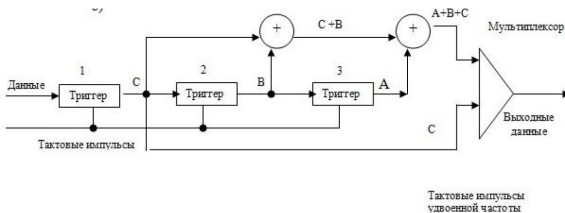
Рис. 5.18. Структурная схема кодера
