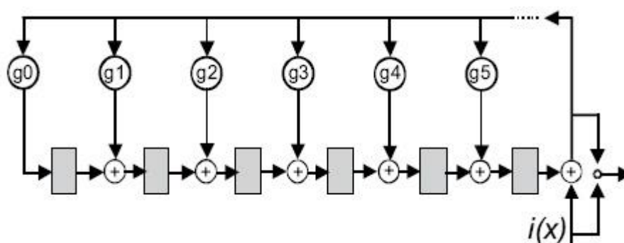
Рис. 3. 41. Схема кодировщика Р-С
