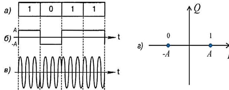
Рис. 1.14. Временная форма и сигнальное созвездие сигнала BPSK: а – цифровое сообщение; б - модулирующий сигнал; в - модулированное ВЧ-колебание; г - сигнальное созвездие
