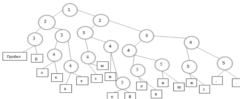
Рис.2.1. Результирующее дерево
