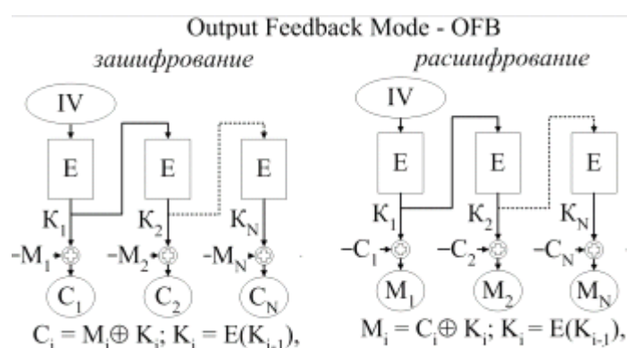
Рис. 2.62. Режим OFB
