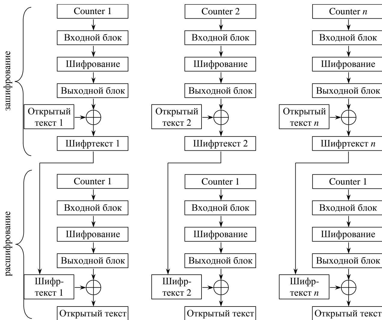
Рис. 2.40. Режим CRT
