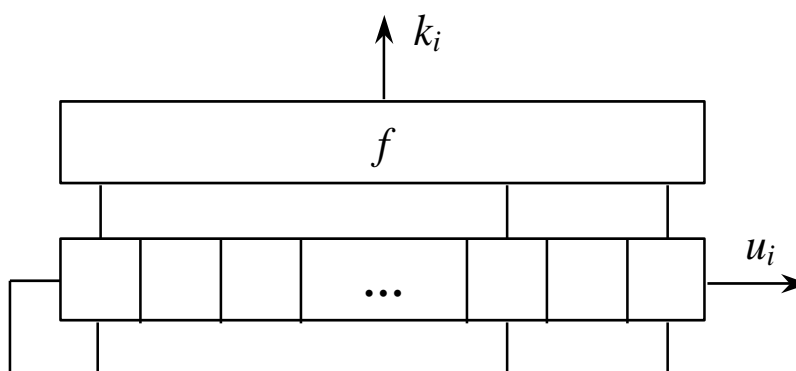
Рис. 2.23. Фильтрующий генератор
