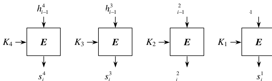
Рис. 3.7. Шифрующее преобразование
