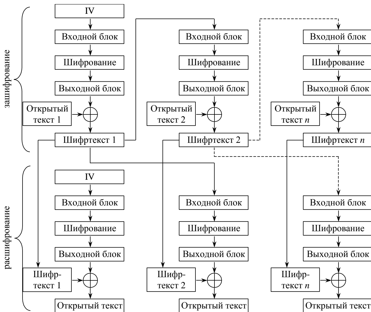
Рис. 2.38. Режим CFB
