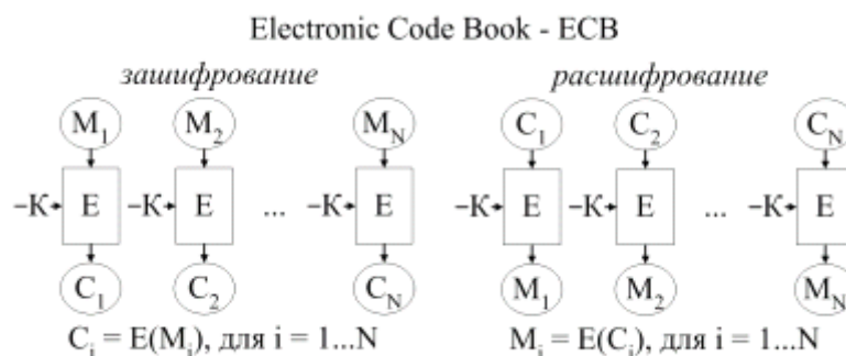
Рис. 2.59. Режим ECB
