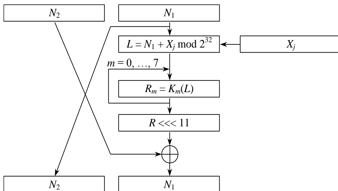
Рис. 2.31. Цикл шифрования
