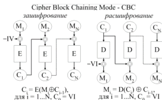
Рис. 2.60. Режим CBC
