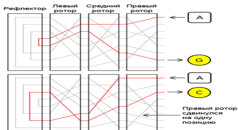
Рис. 1.24. Схема шифрования
