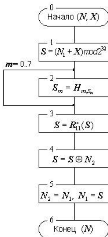
Рис. 2.42. Схема основного шага криптопреобразования алгоритма ГОСТ 28147-89
