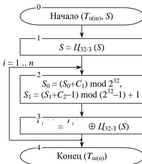
Рис. 2.5. Алгоритм зашифрования (расшифрования) данных в режиме гаммирования
