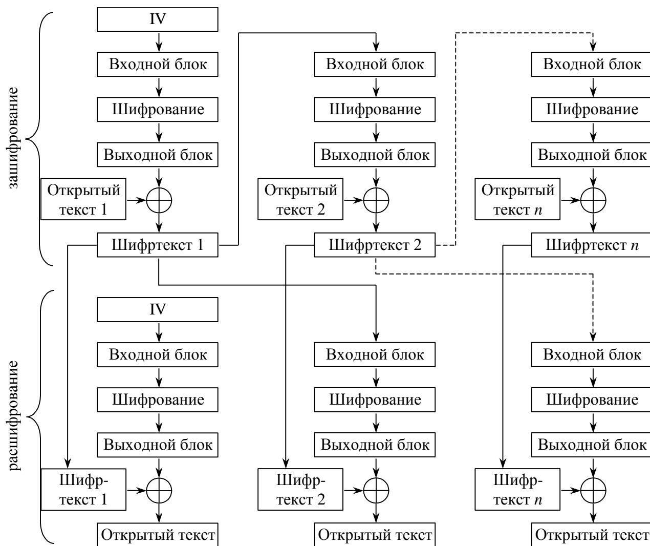
Рис. 2.38. Режим CFB
