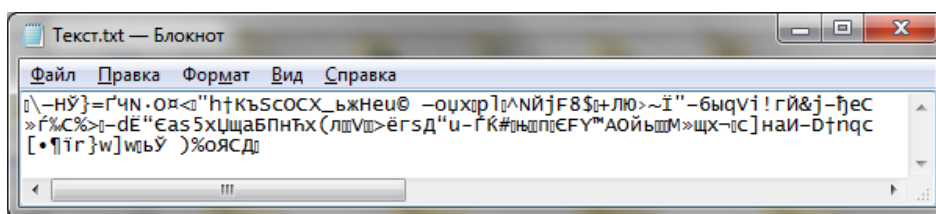
Рис. 2.67. Зашифрованный текст
