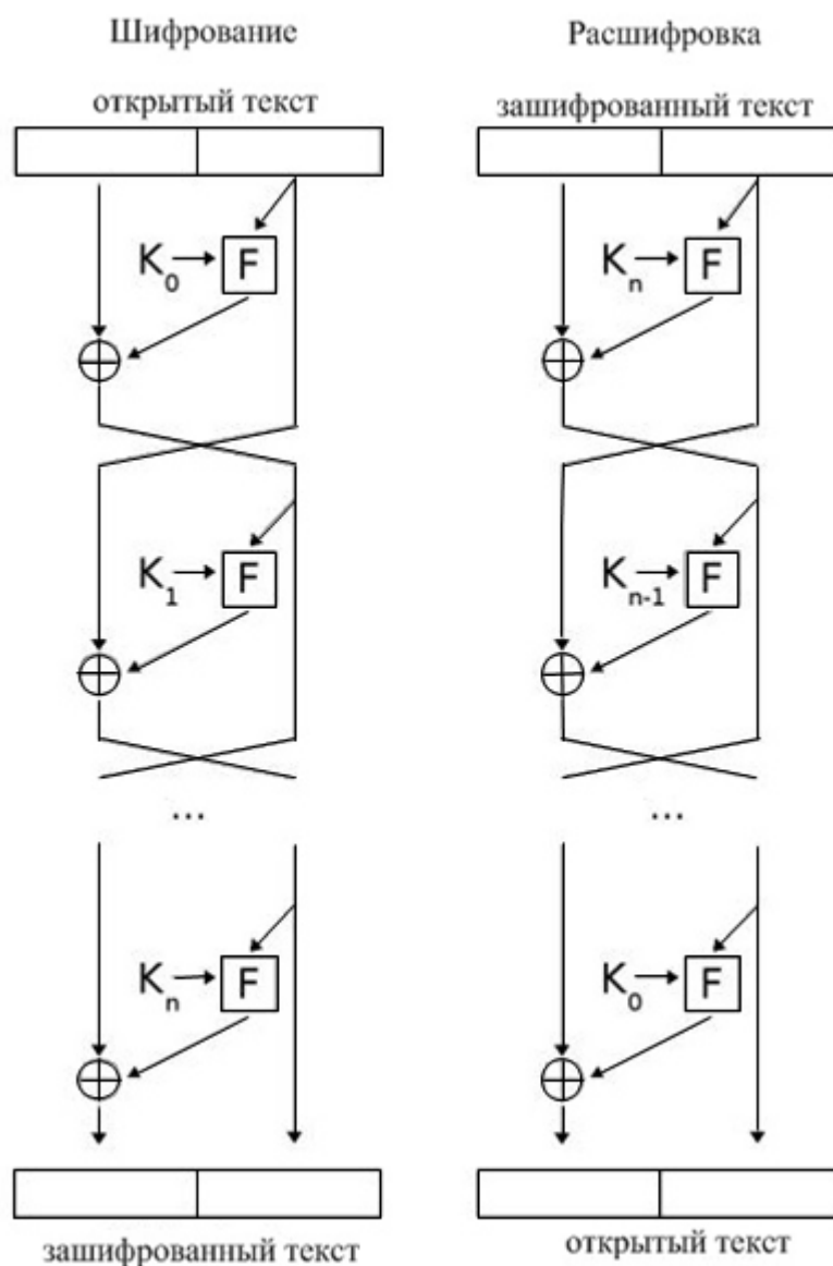
Рис. 2.41. Сеть Фейстеля
