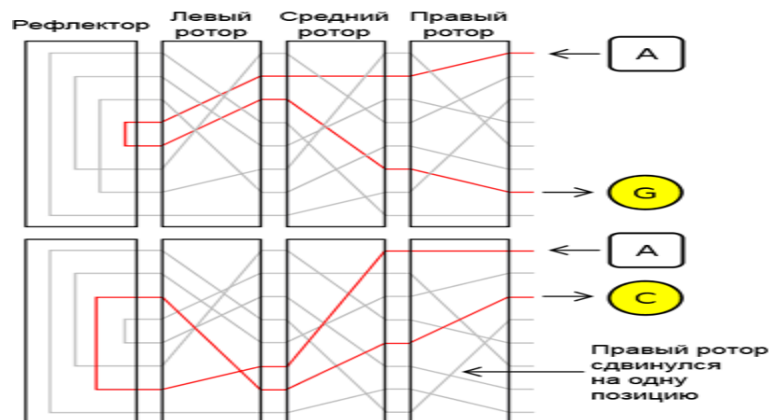
Рис. 1.24. Схема шифрования
