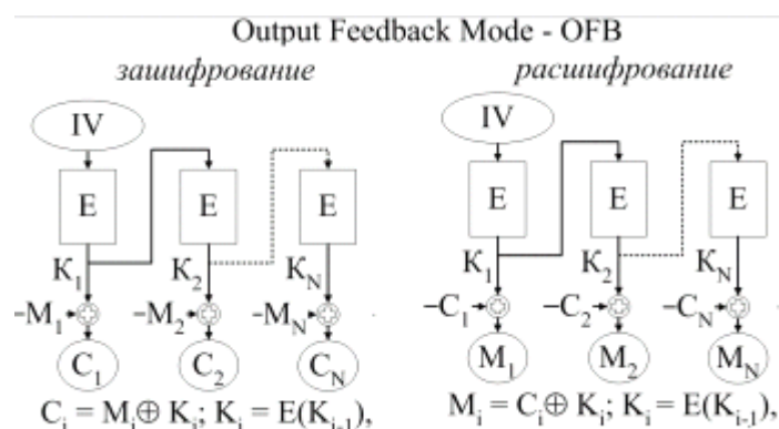
Рис. 2.62. Режим OFB
