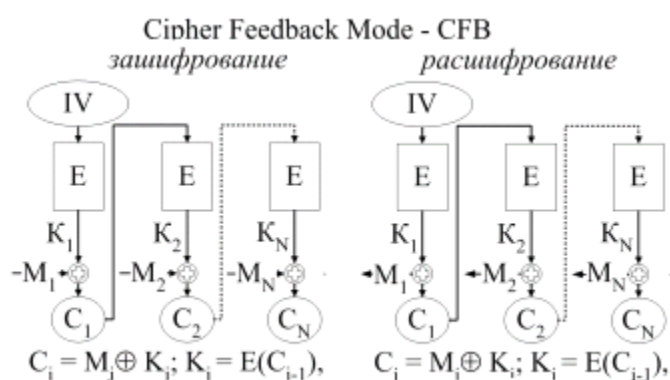
Рис. 2.61. Режим CFB
