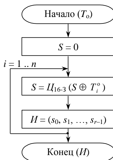
Рис. 2.7. Алгоритм выработки имитовставки для массива данных
