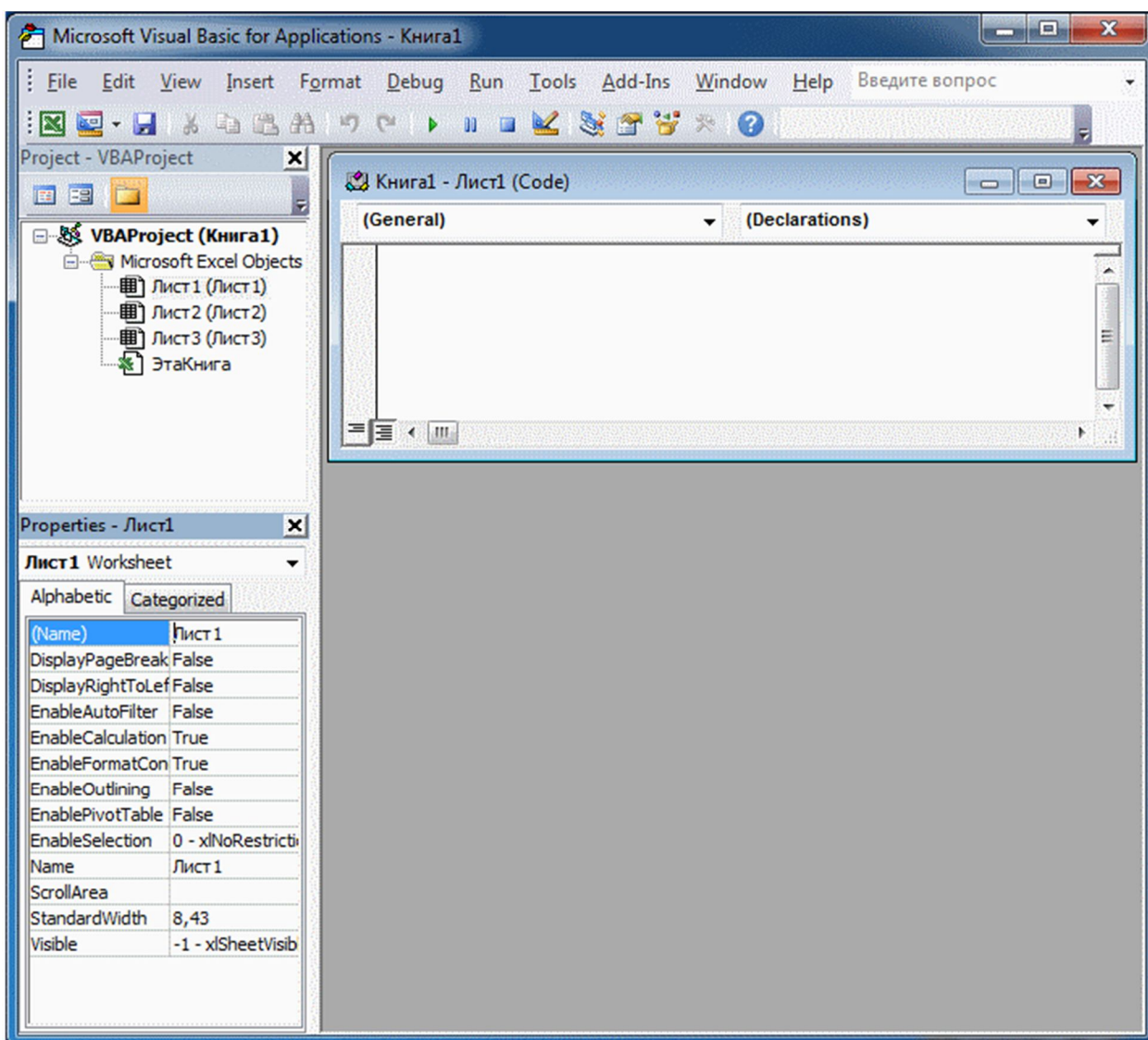
Рис. 4 Редактор VBA
