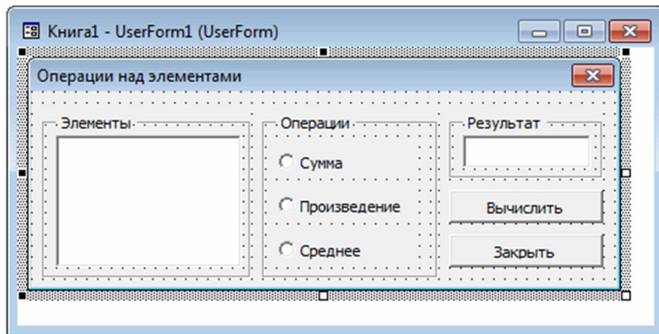
Рис. 14 Объект UserForm
