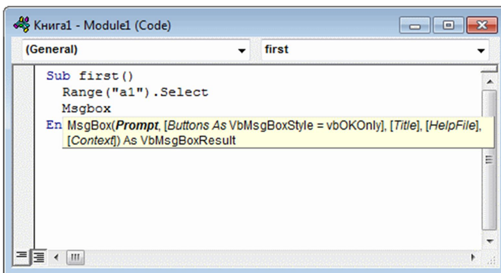
Рис. 9 Отображаемые сведения о вводимой процедуре
