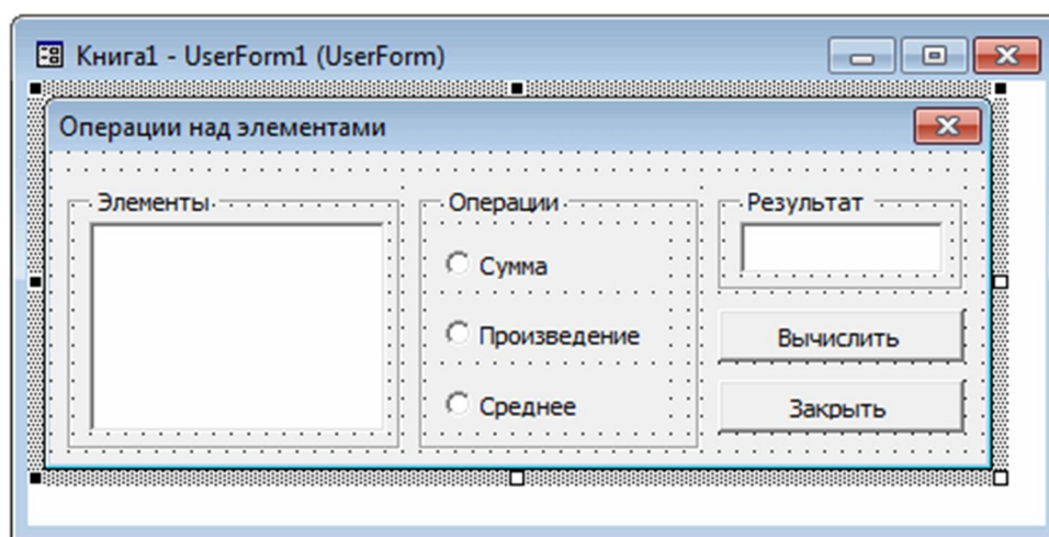
Рис. 14 Объект UserForm
