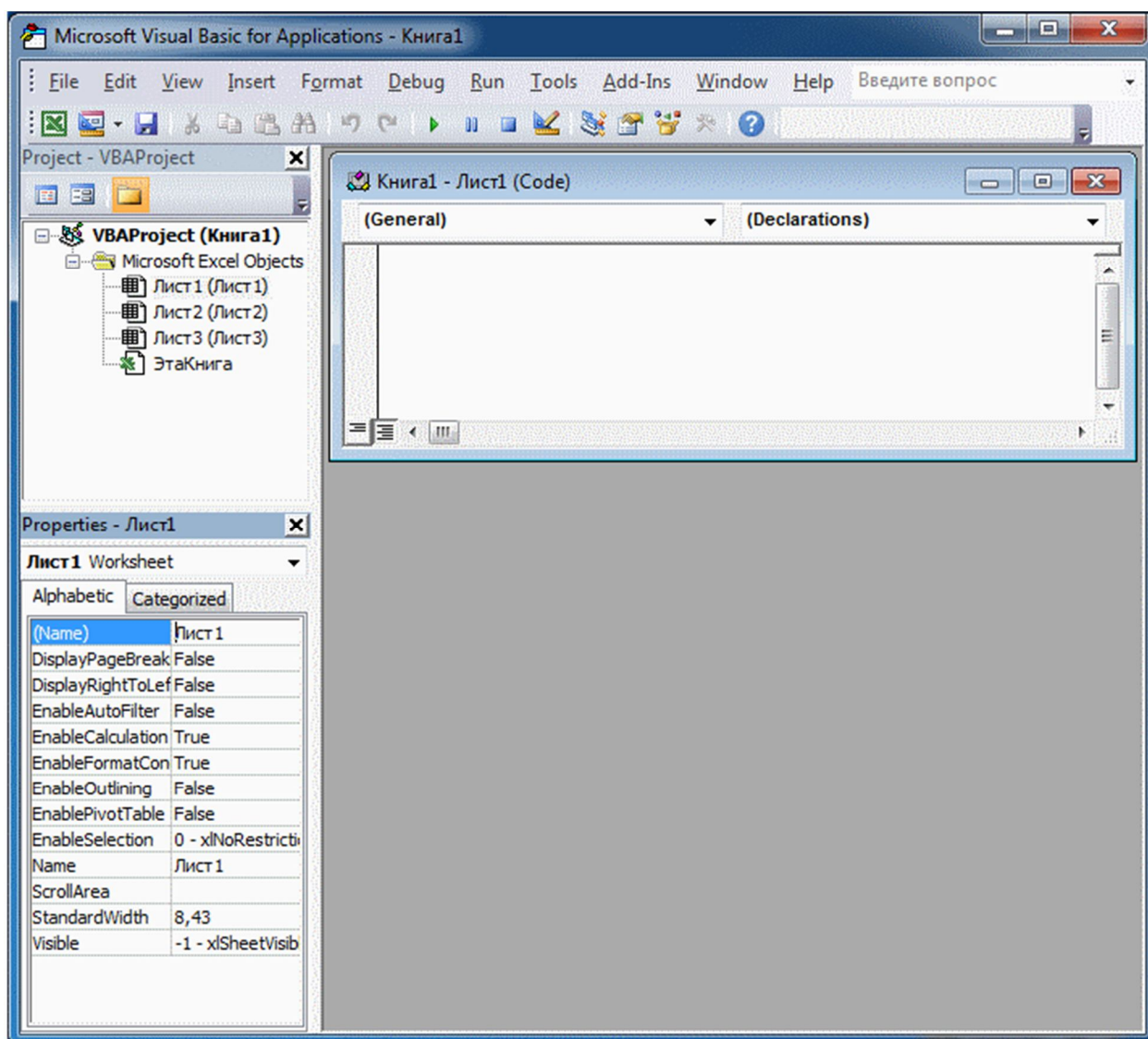
Рис. 4 Редактор VBA
