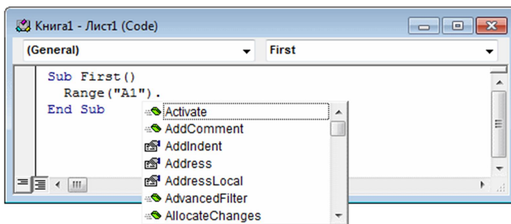
Рис. 8 Список компонентов
