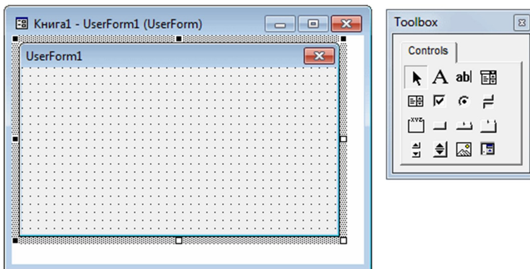
Рис. 13 Объект UserForm
