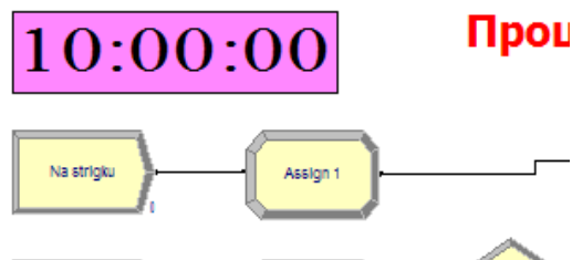
Рис. 4.18. Добавление часов
