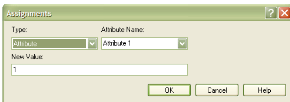
Рис. 3.10. Добавление атрибута
