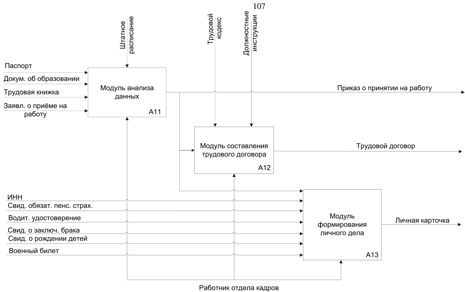
Приложение В Диаграмма А1 «Подсистема приёма сотрудников на работу» (обязательное)
