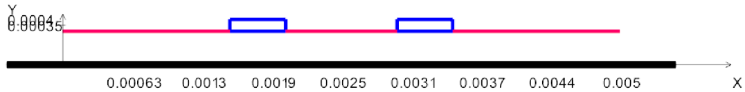
Рисунок 1.8 – Вид связанной микропослосковой линии в системе TALGAT (синий цвет – проводниковые границы, красный – диэлектрические границы)
