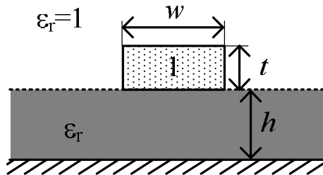
Рисунок 1.20 – Поперечное сечение микрополосковой линии
