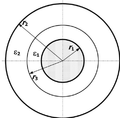
Рис. 2.9 – Кабель с градированной изоляцией Радиус оболочки r_2 в этом случае может быть найден из равенства
