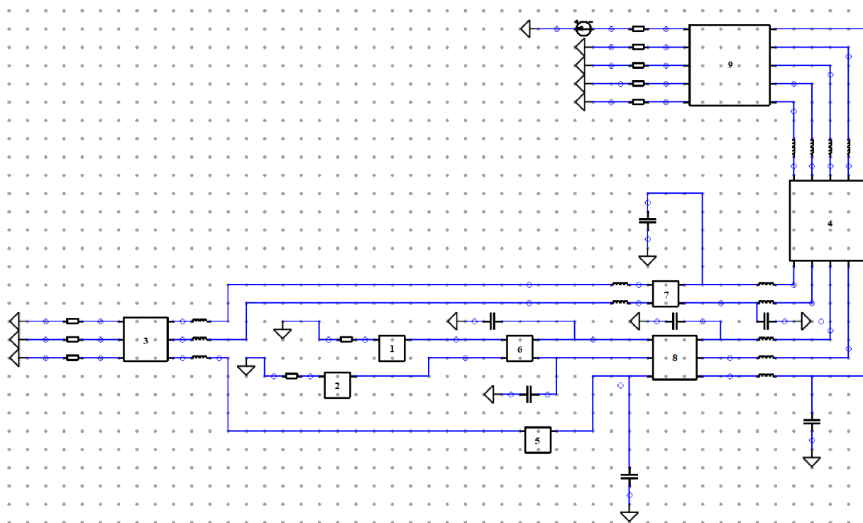
Рисунок 2.7 – Принципиальная схема
