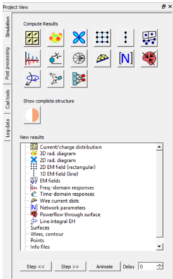
Рисунок 1.36 – Постобработка вычислений
