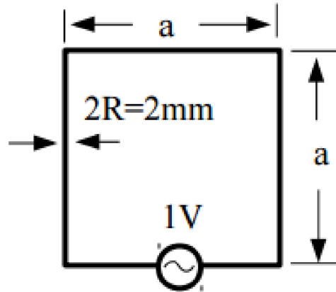
Рисунок 2.14 – Параметры контурной антенны
