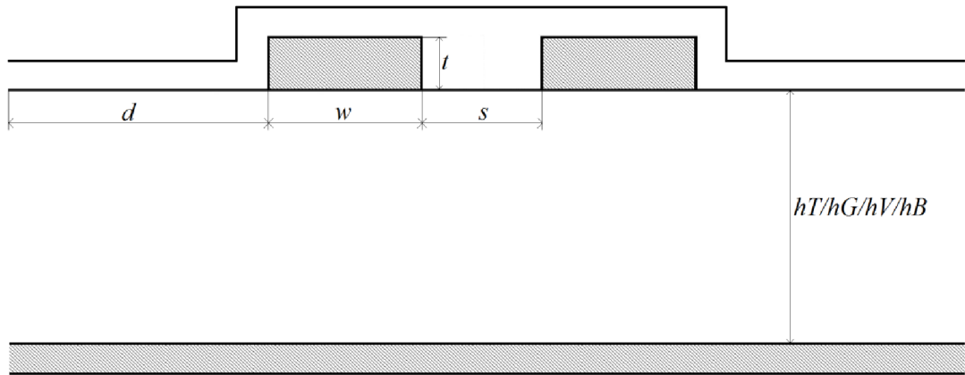
Рисунок 2.2 – Поперечное сечение линии передачи
