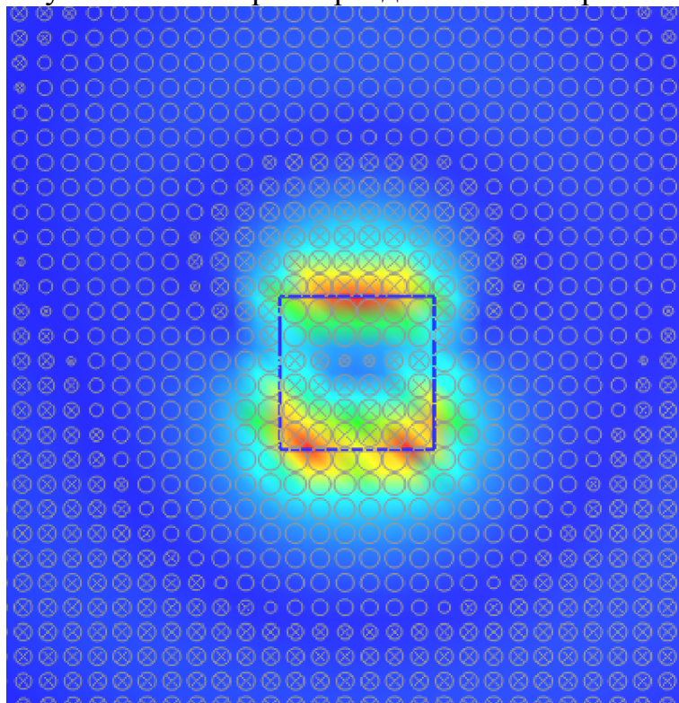
Рисунок 2.28 – Распределение поля H на частоте 1ГГц
