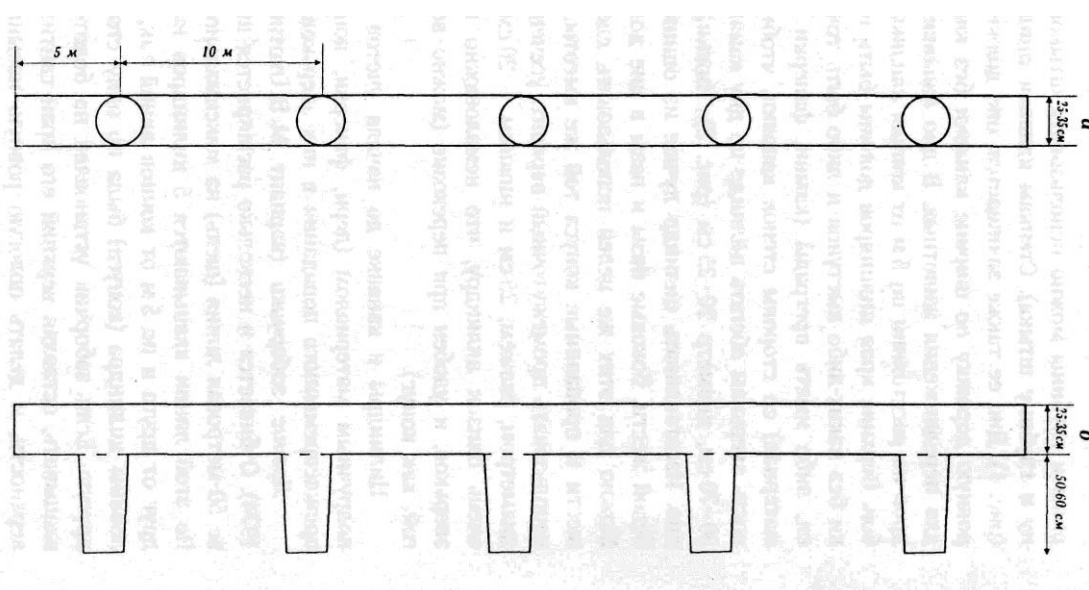
Рис. 4. Схема строения ловчей канавы
