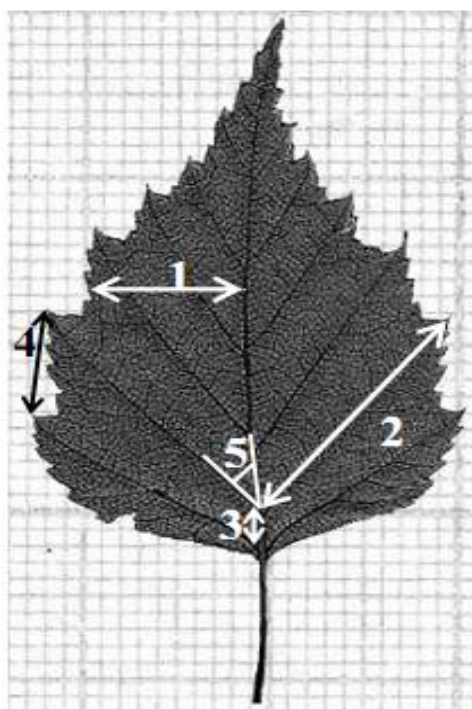
Рис. 6. Схема промеров листа березы повислой Математическая обработка результатов Мерные признаки
