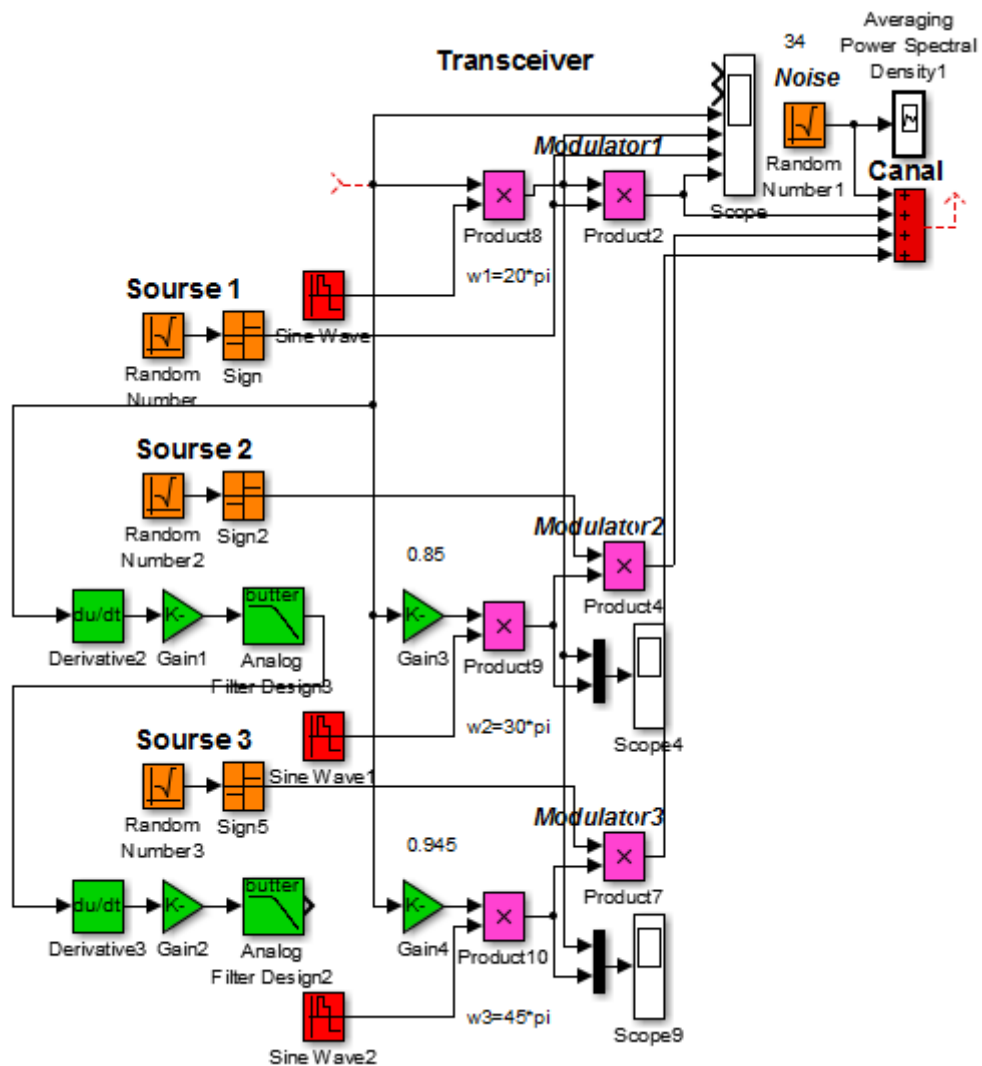
Рисунок 3.3 – Функциональная схема передатчика
