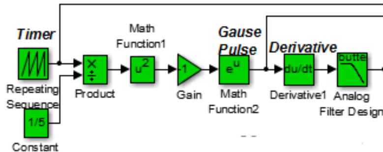
Рисунок 3.2 – Функциональная схема генератора импульсов Гаусса
