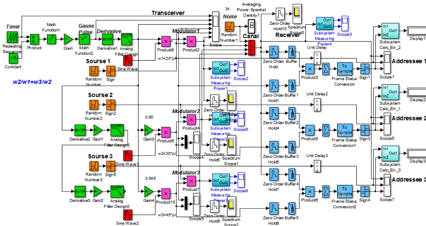
Рисунок 3.1 - Функциональная модель 3-х канальной сверхширокополосной радиосвязи на основе на основе импульсов Гаусса и частотного разделения каналов
