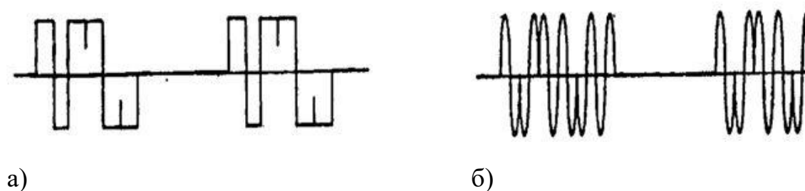
Рисунок 3 — Кодированные сигналы на основе видеоимпульсов (а) и однопериодных радиоимпульсов (б)
