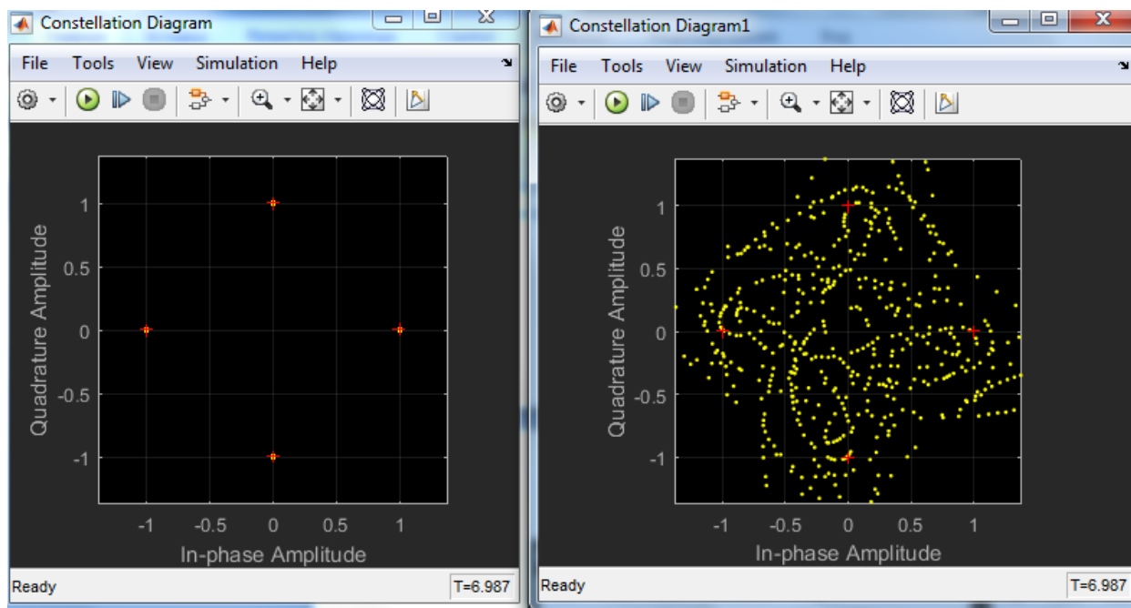
Рис. 7.10. Сравнение передаваемого созвездия и принятого, при отношении С/Ш – 20 Дб.
