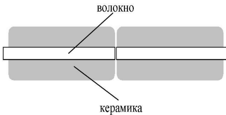
Рис. 4.27. Стык оптоволоконна
