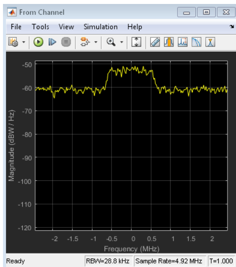
Рис. 7.26. Спектр принимаемого мобильной станцией сигнала после прохождения через канал
