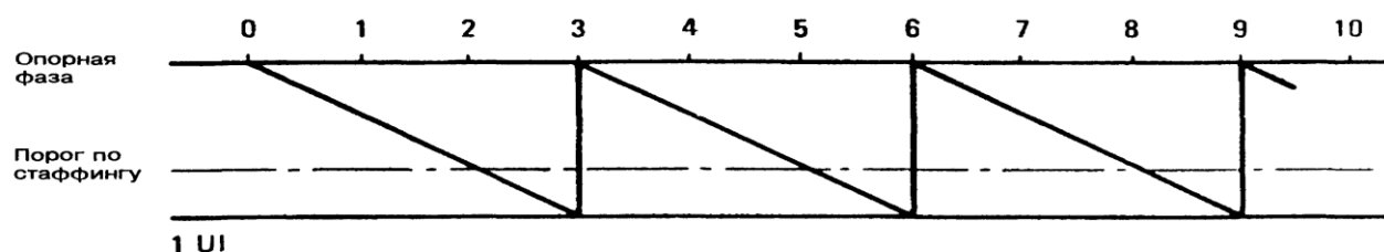
Рис. 1.26. Стаффинг с отношением 5 = 1/3
