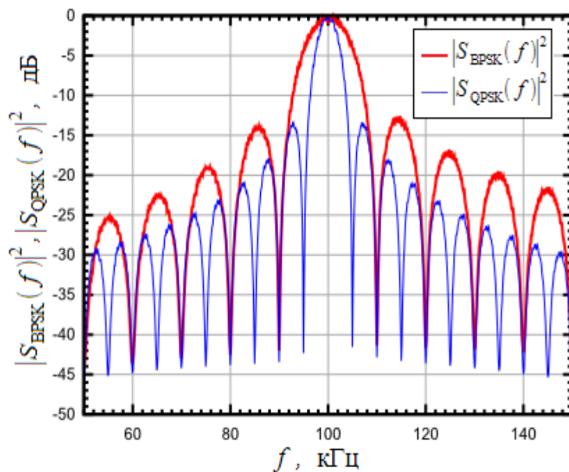
Рис. П1.36. Спектр QPSK сигнала.
