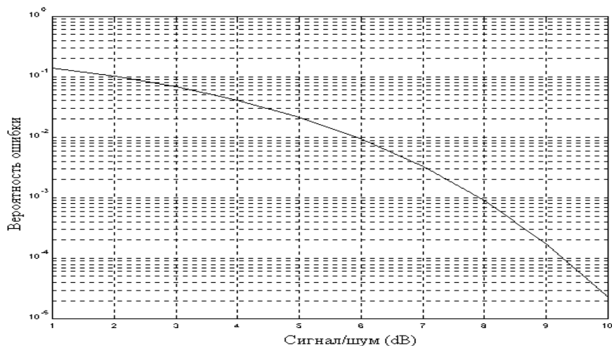
Рис. П1.13. График зависимости вероятности ошибки GMSK в зависимости от отношения сигнал/шум на входе решающего устройства
