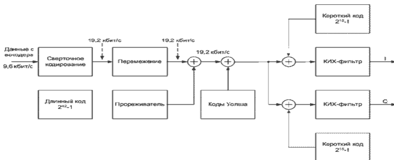
Рис. 7.17. Схема кодирования в обратном канале.
