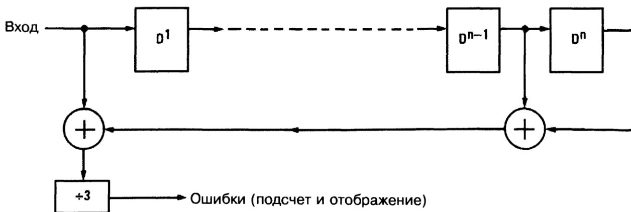
Рис. 1.13. Анализатор ПСП без обратной связи
