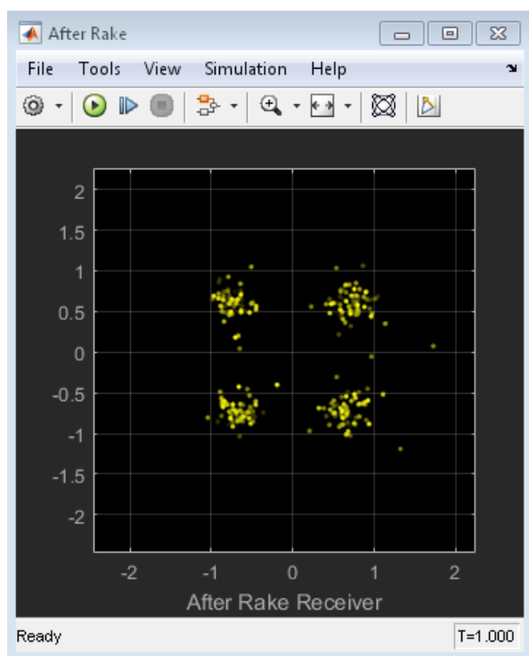
Рис. 7.29. Сигнал, декодированный мобильной станцией, на I-Q диаграмме.
