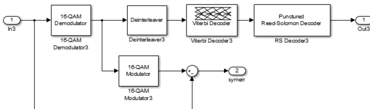
Рисунок 7.95 – Состав блока демодулятора «16QAM 1/2»
