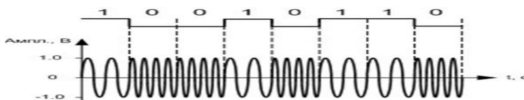
Рис. П1.1. Частотная манипуляция
