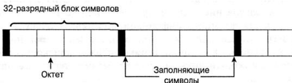
Рис. 7.47. Скрэмблированный PSDU в технологии FHSS
