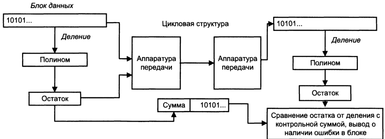
Рис. 1.17. Алгоритм использования избыточного циклового кода
