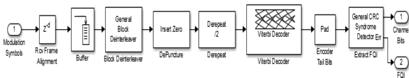
Рис. 7.23. Модель декодера.
