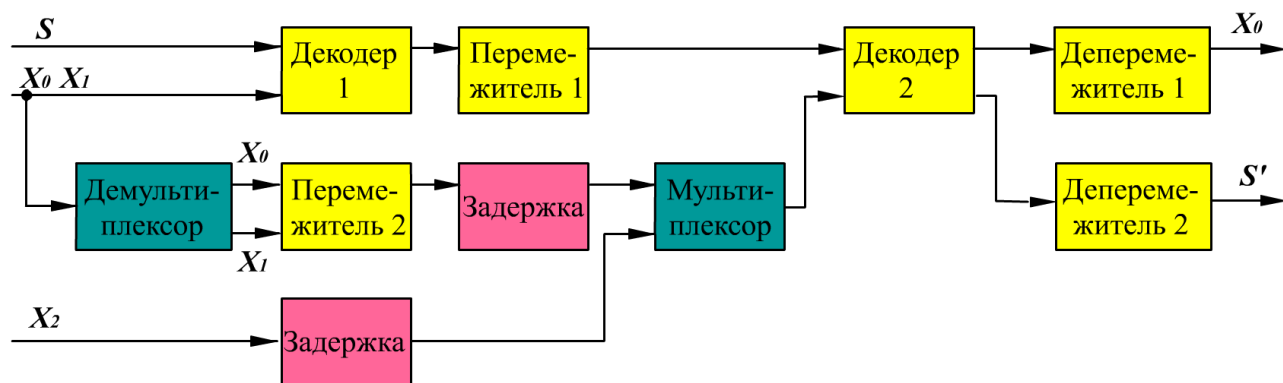
Рисунок П1.75. Структурная схема одной итерации турбо-декодера при двухкаскадном кодировании
