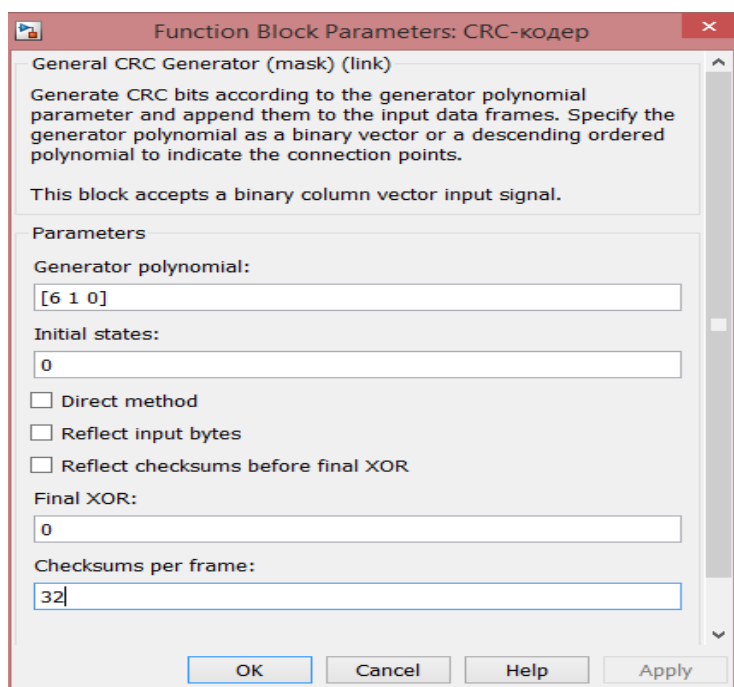
Рис. П1.71. Параметры блока CRC-кодер
