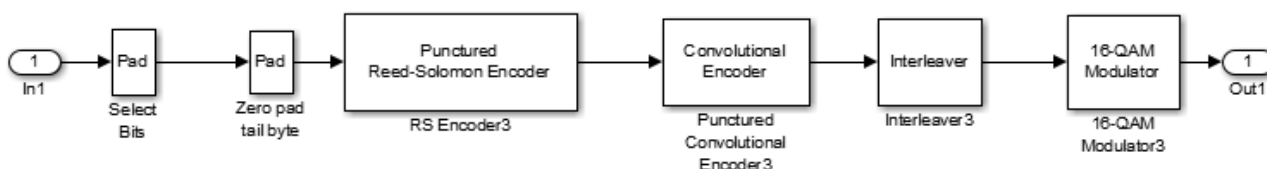
Рисунок 7.82 – Состав блока модулятора «16QAM 1/2»
