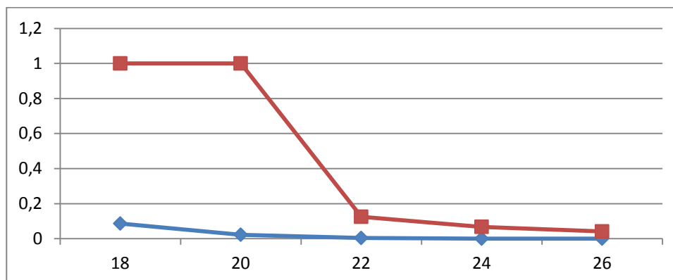
Рис. П1.9. Зависимость вероятности ошибки от отношения сигнал/шум
