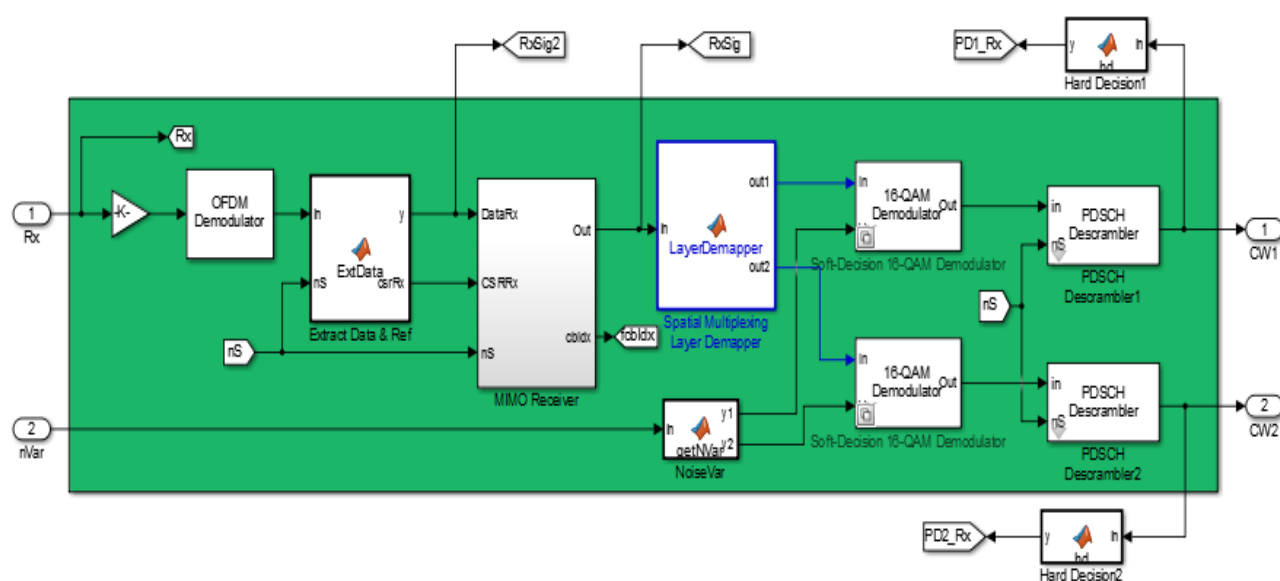
Рис. 7.138. Параллельные потоки-ОДПФ-демодуляция
