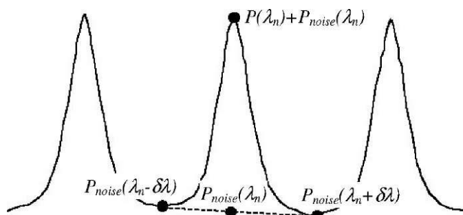
Рис. 4.81. К оценке OSNR по реальной спектральной характеристике группового оптического сигнала
