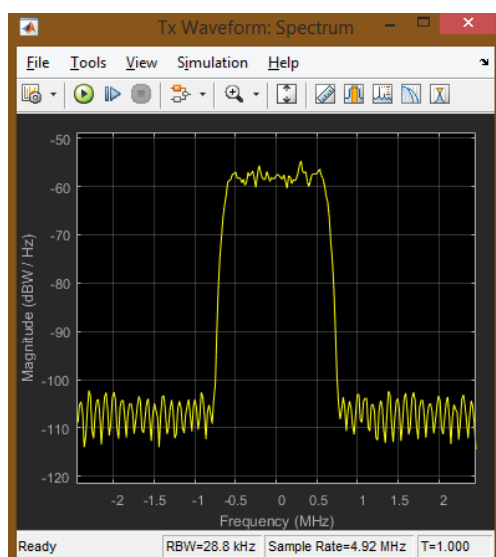
Рис. 7.30. Спектр сигнала сгенерированного базовой станцией
