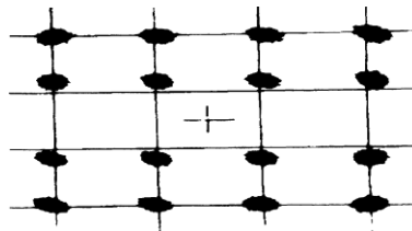
Рис. 2.14. Несбалансированность по амплитуде сигнала на диаграмме состояний
