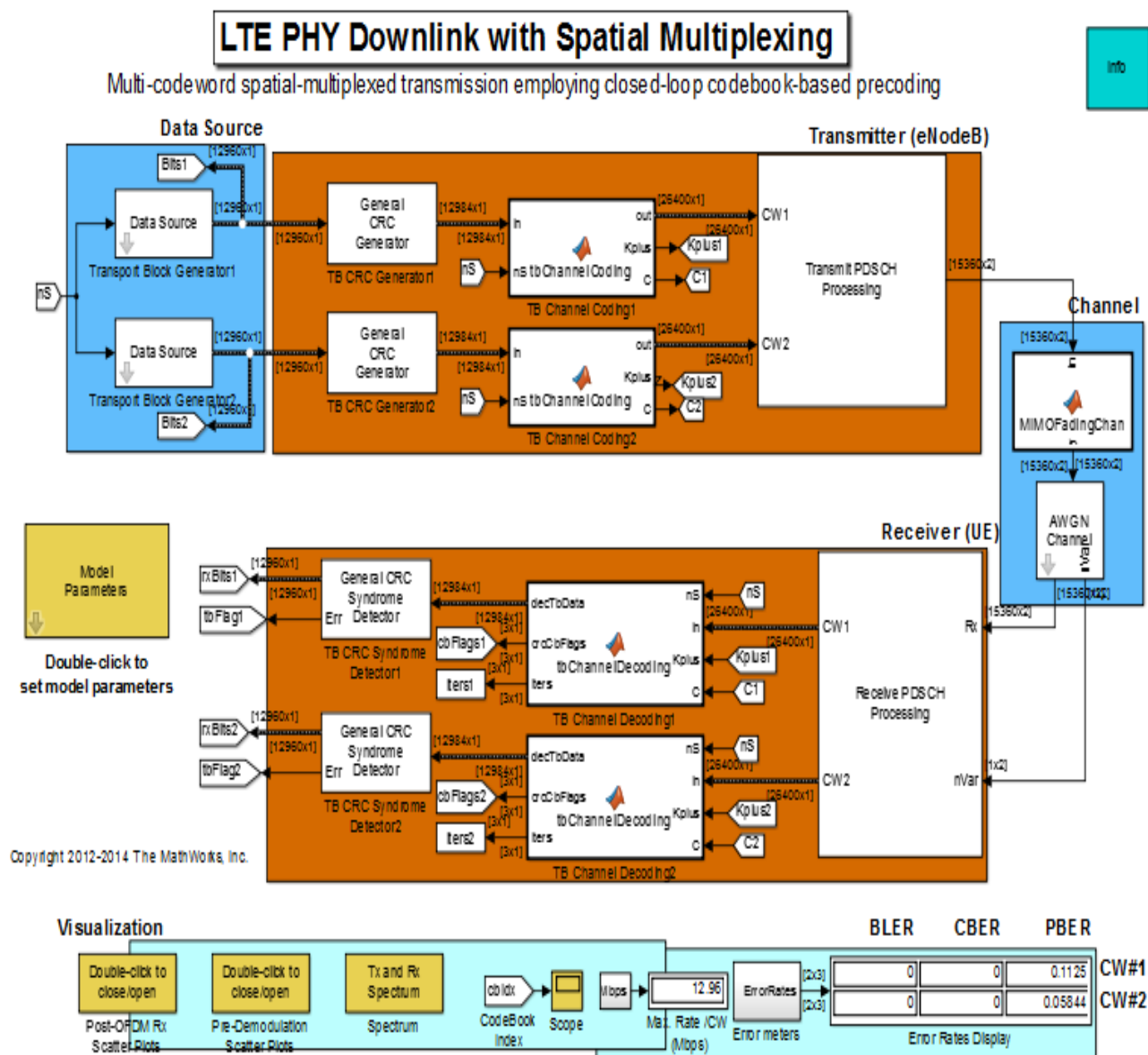
Рис. 7.157. Схема канала Downlink
