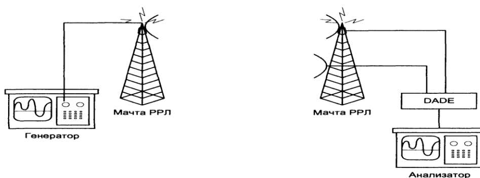
Рис. 2.37. Измерения DADE
