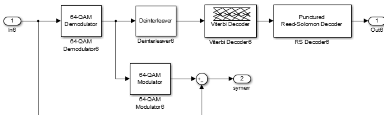
Рисунок 7.98 – Состав блока демодулятора «64QAM 3/4»
