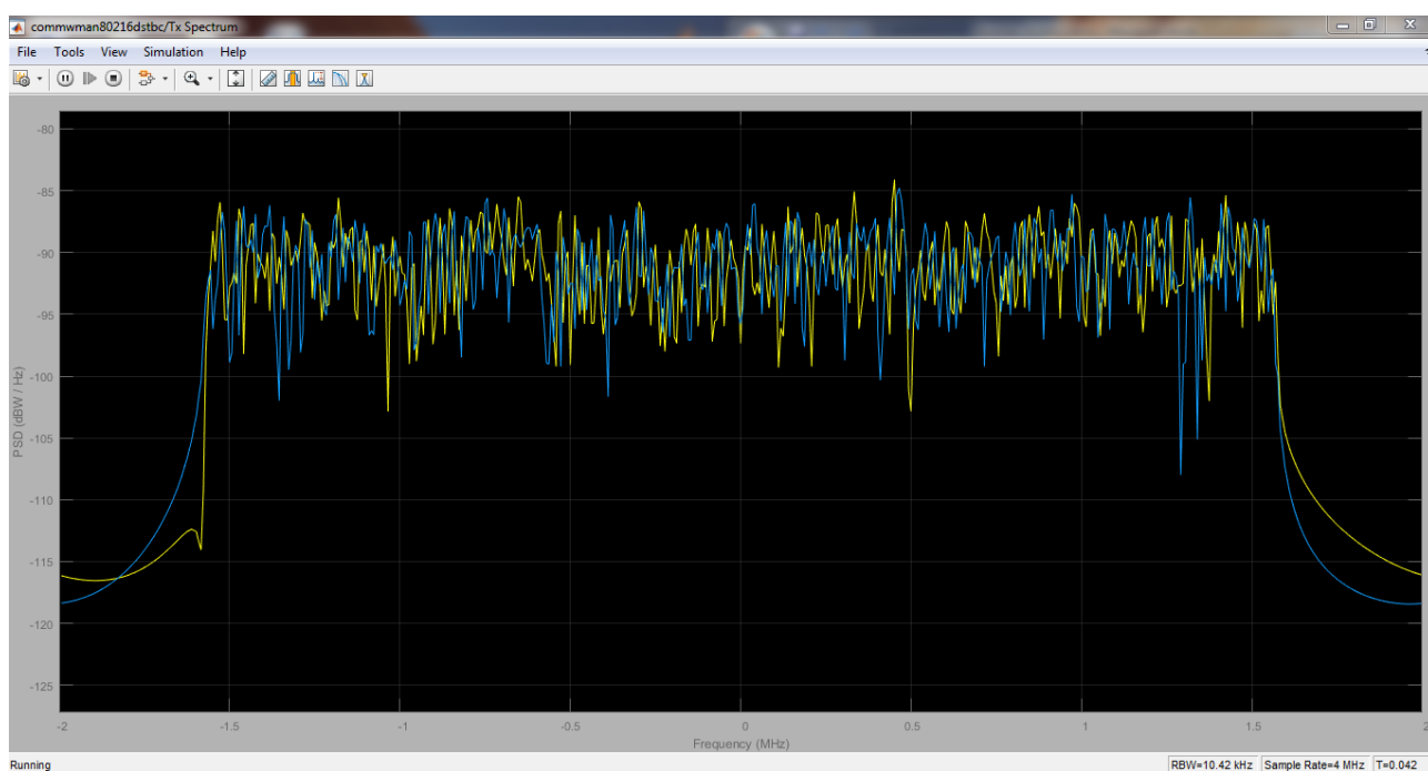
Рисунок 7.108 – Спектр передаваемых сигналов, поступающих на соответствующую передающую антенну
