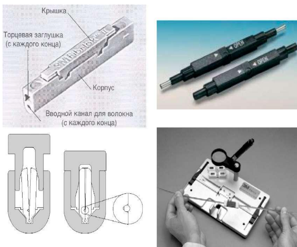
Рис. 4.29. Механический соединитель
