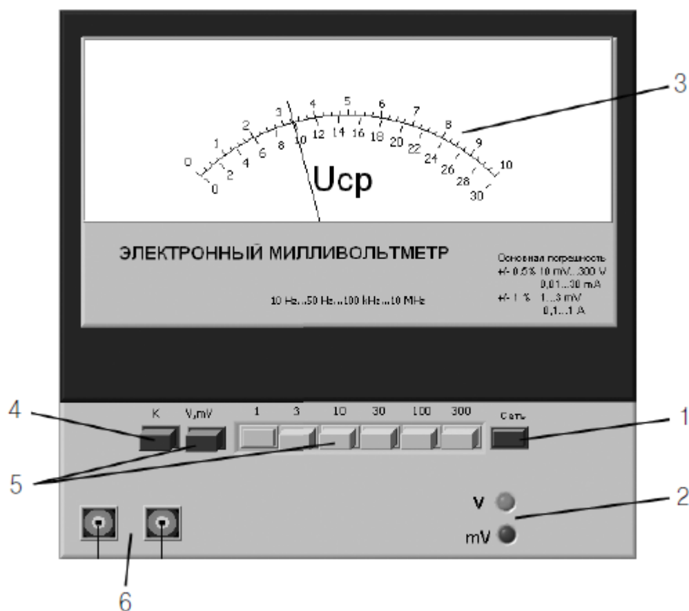
Рис. 5.11. Внешний вид модели электронного аналогового милливольтметра средневыврямленного значения
