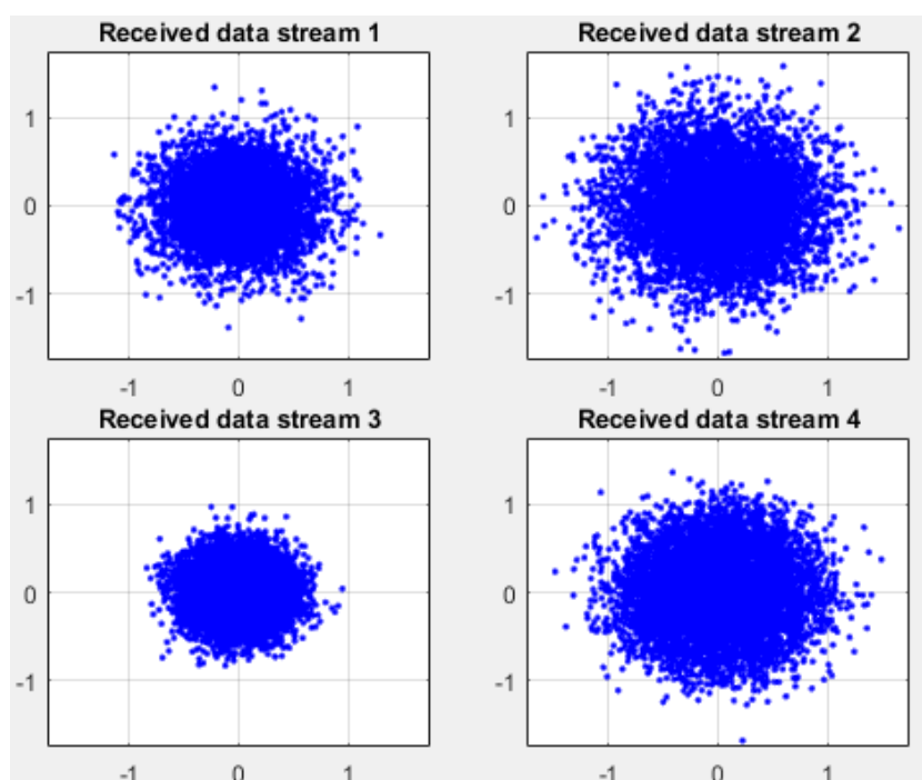
Рис. 7.147. Диаграмма созвездий принятого сигнала для каждой из антенн ММО
