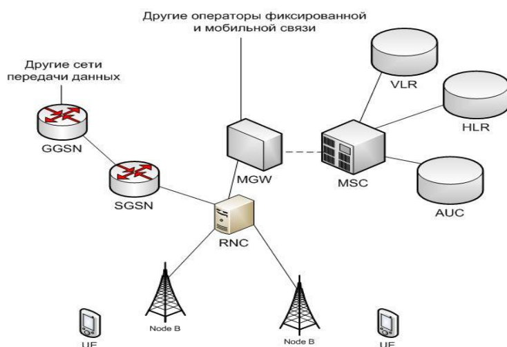
Рис. 7.119. Структура сети стандарта 3G (UMTS)
