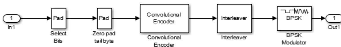
Рисунок 7.79 – Состав блока модулятора «BPSK 1/2»
