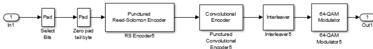
Рисунок 7.84 – Состав блока модулятора «64QAM 2/3»
