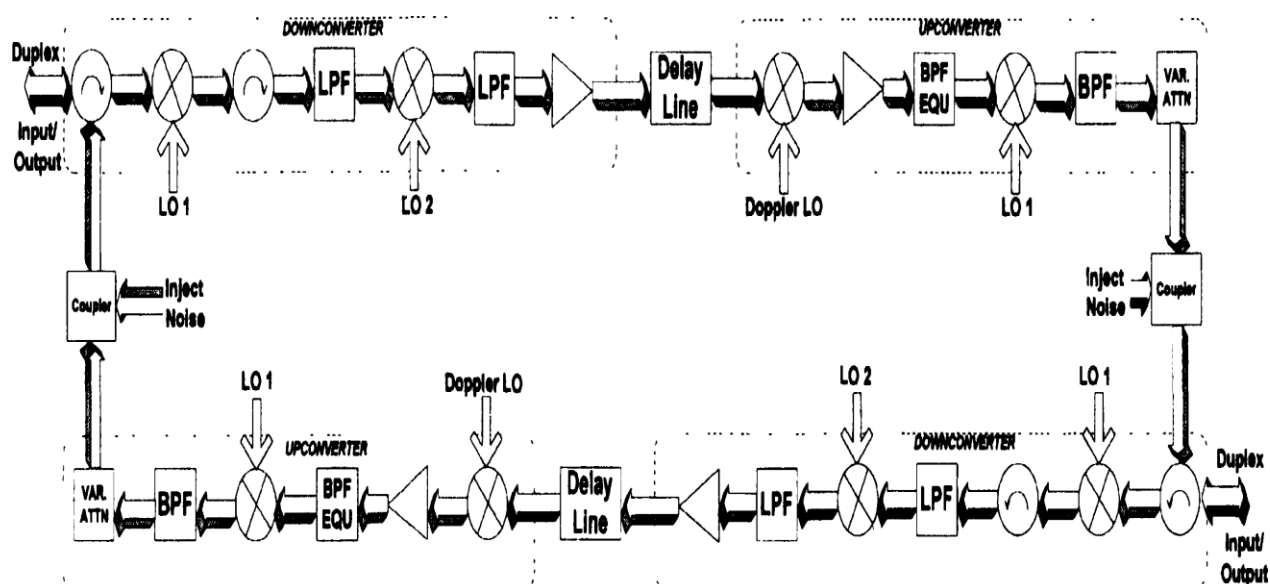
Рис. 2.41. Схема имитатора спутникового канала SLE-250/SLE-500
