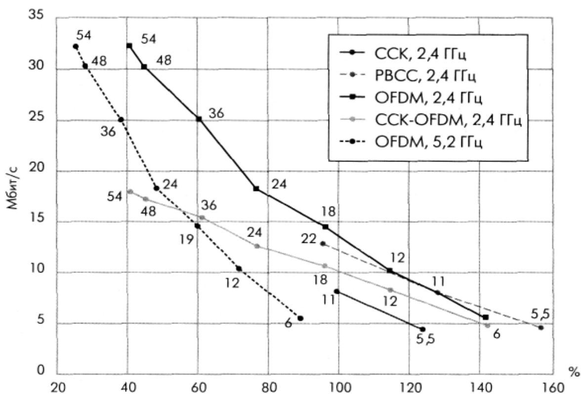
Рис. 7.57. Зависимость скорости передачи от расстояния для различных технологий передачи. Расстояние приведено в процентах, 100% - дальность передачи с модуляцией ССК на скорости 11 Мбит/с
