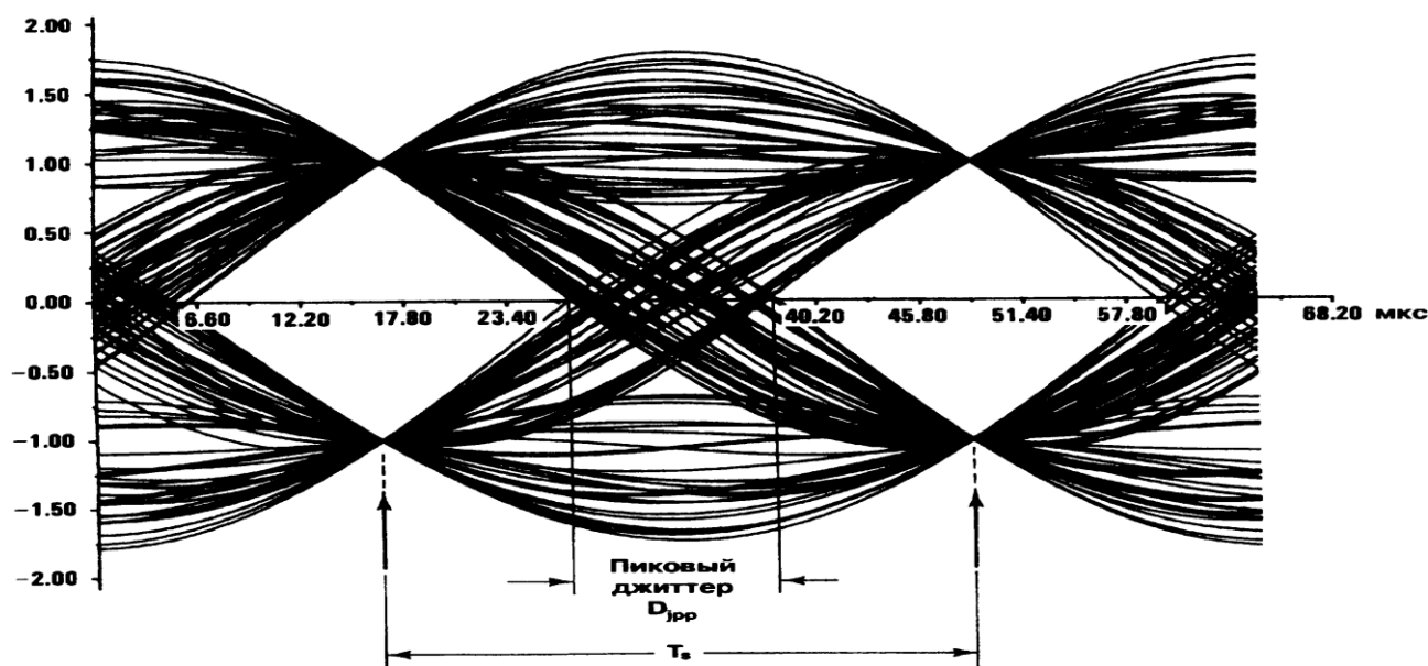
Рис. 1.3. Глазковая диаграмма цифрового сигнала, проходящего через фильтр с коэффициентом ограничения спектра a=0,3 (компьютерная имитация)
