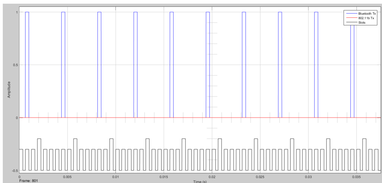
Рис. 7.62. Временная диаграмма Bluetooth без мешающего сигнала 802.11
