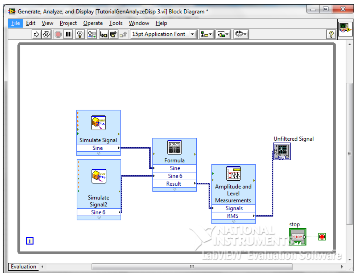
Рис. 5.3. Блок-диаграмма
