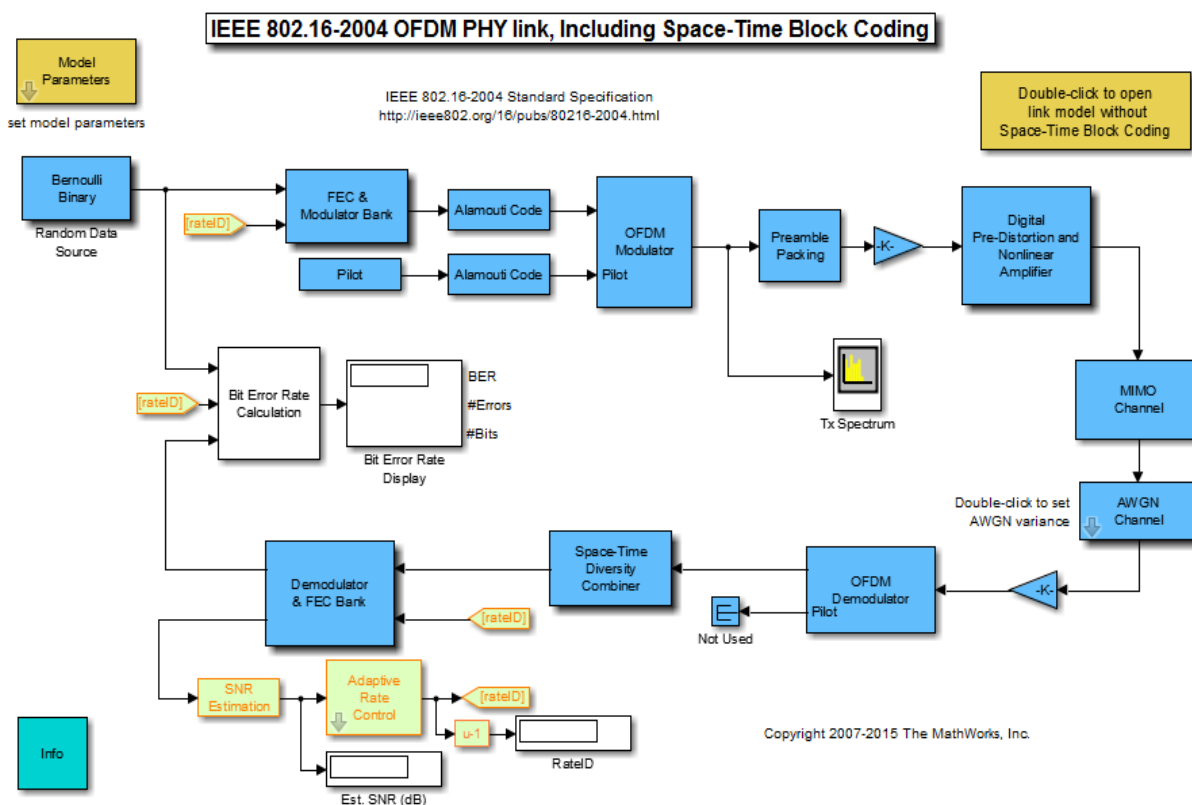
Рисунок 7.75 – Модель IEEE 802.16-2004 OFDM в MATLAB 2015b
