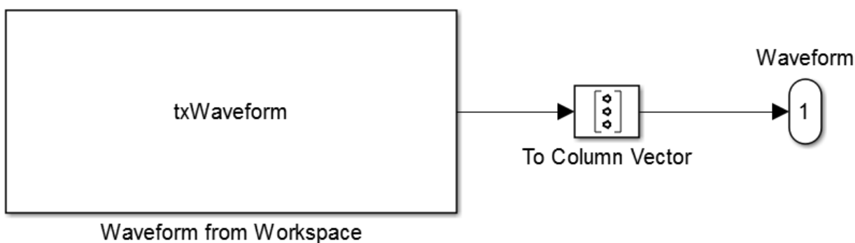
Рис. 7.20. Модель передатчика
