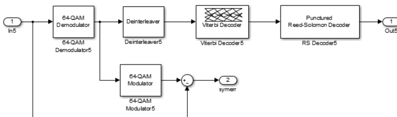
Рисунок 7.97 – Состав блока демодулятора «64QAM 2/3»
