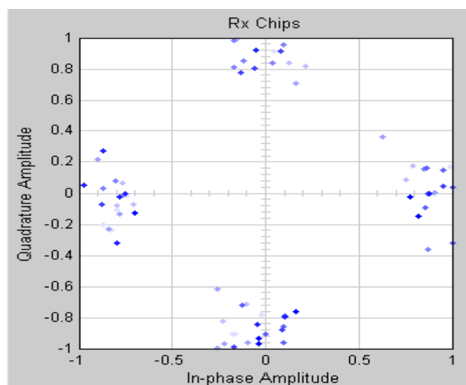
Рис. 7.63. Диаграмма созвездий для скорости передачи 11 Мбит/с
