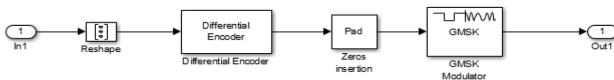
Рис. 7.5. Схема модулятора
