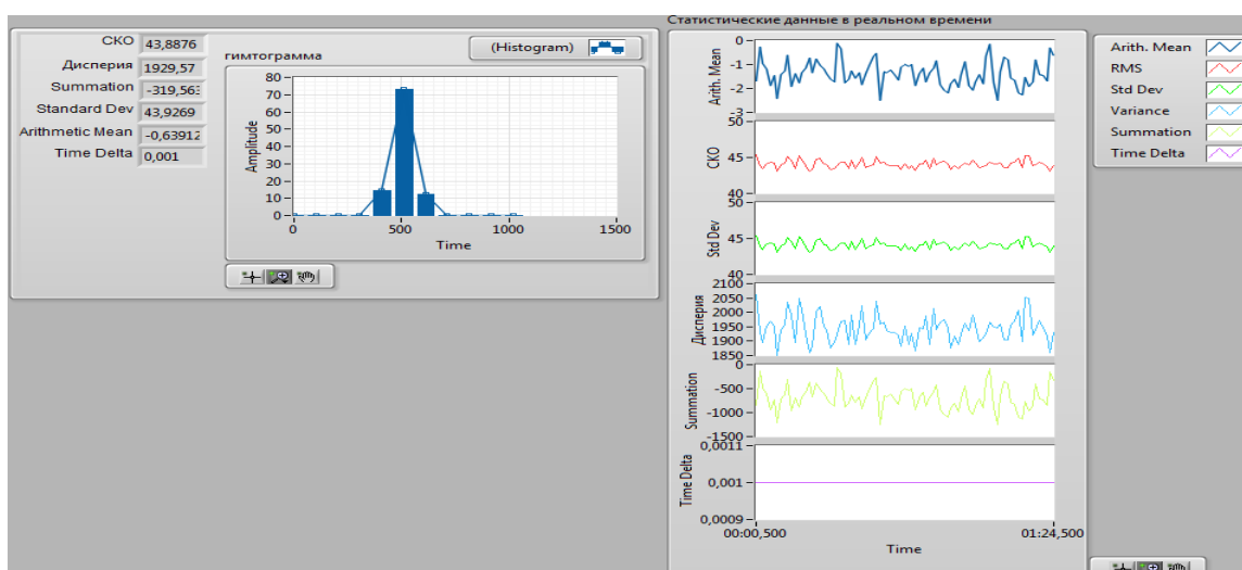
Рис. П2.10. Лицевая панель статистической обработки сигналов.
