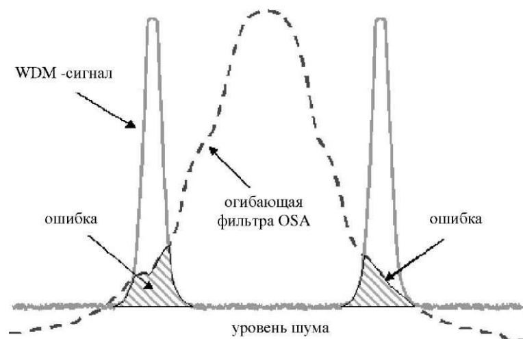
Рис. 4.77. WDM сигнал
