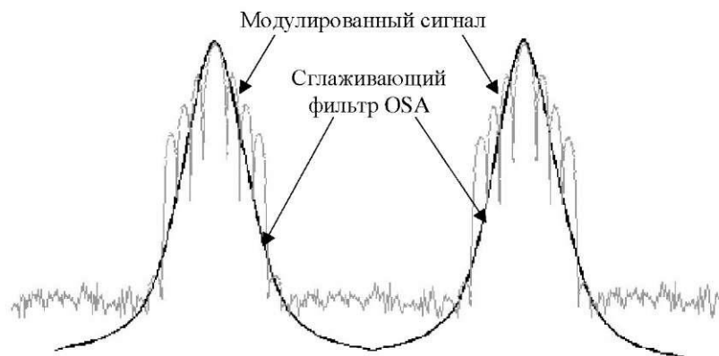
Рис. 4.76. Модулированный сигнал
