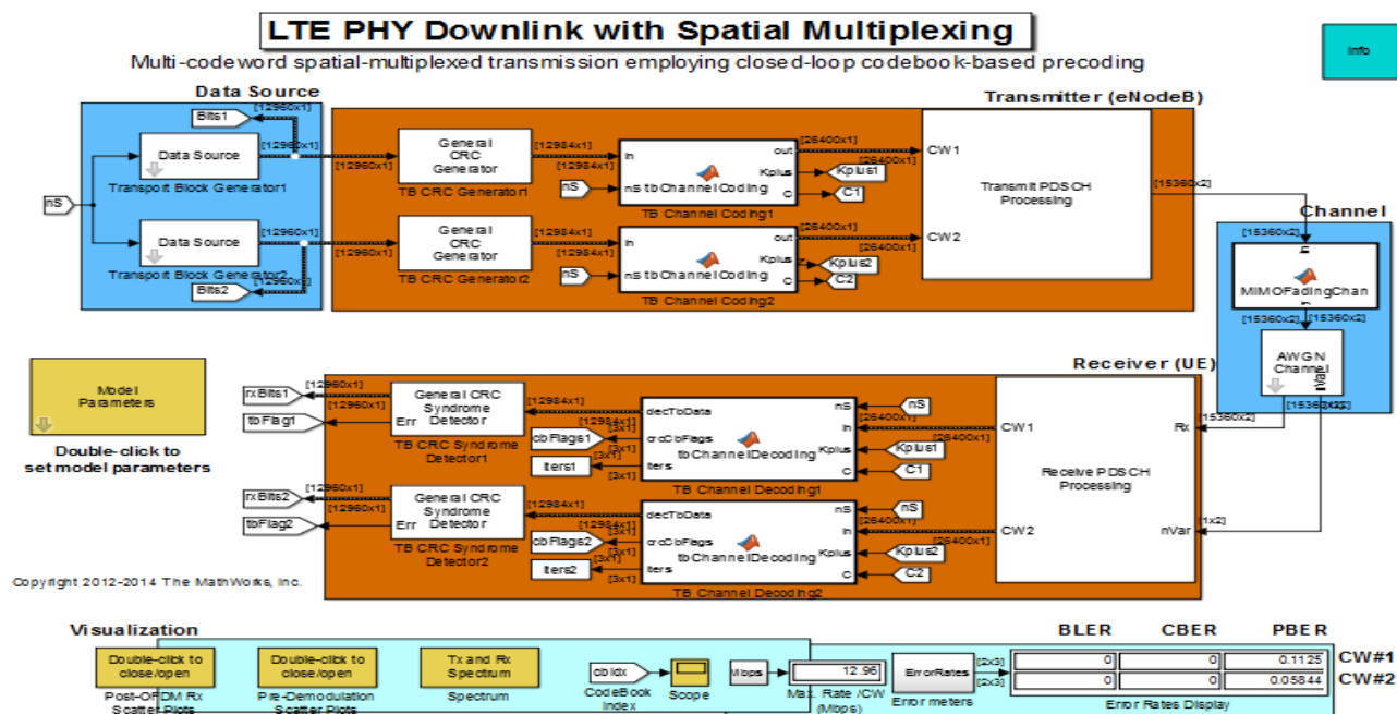
Рис. 7.129. Канал Downlink LTE Simulink MATLAB 2015b
