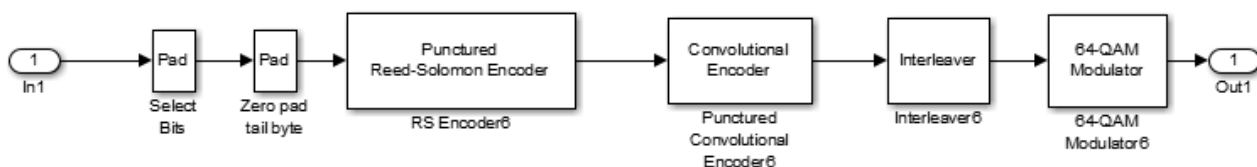
Рисунок 7.85 – Состав блока модулятора «64QAM 3/4»
