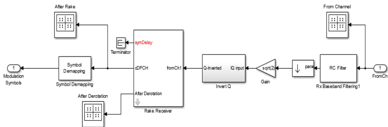
Рис. 7.21. Модель приемника
