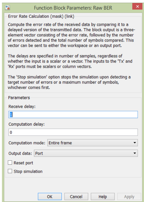
Рис. 7.81. Параметры блока RawBER
