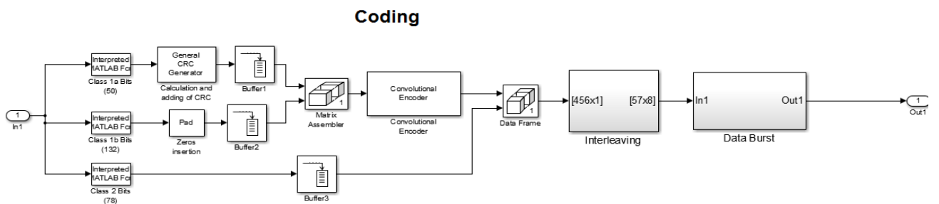
Рис. 7.4. Схема кодера
