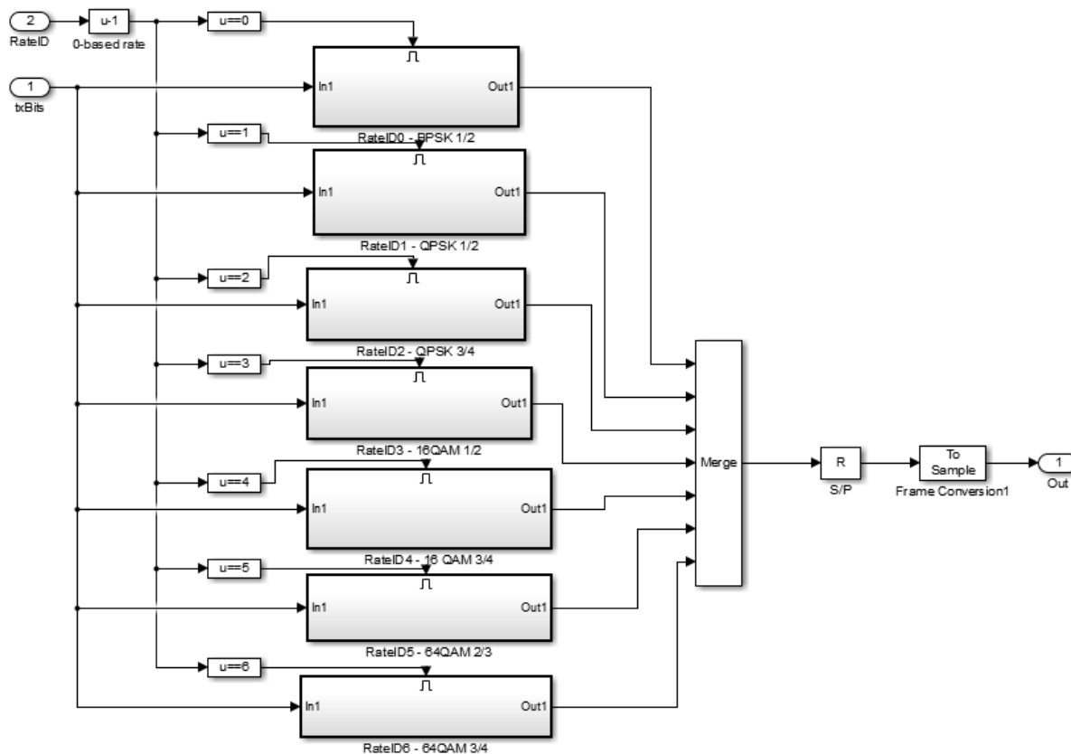
Рисунок 7.78 – Состав блока «FEC & Modulator Bank»
