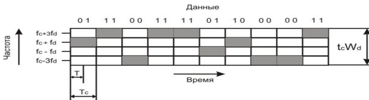
Рис. П1.2. Использование частоты схемой MFSK ( M = 4 )
