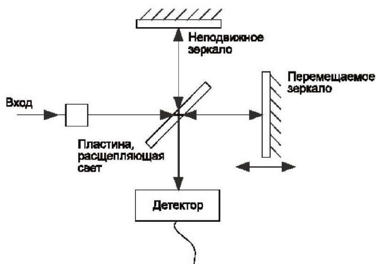
Рис. 4.65. Интерферометрический метод
