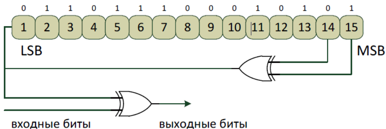
Рисунок 7.71 – Схема скремблера
