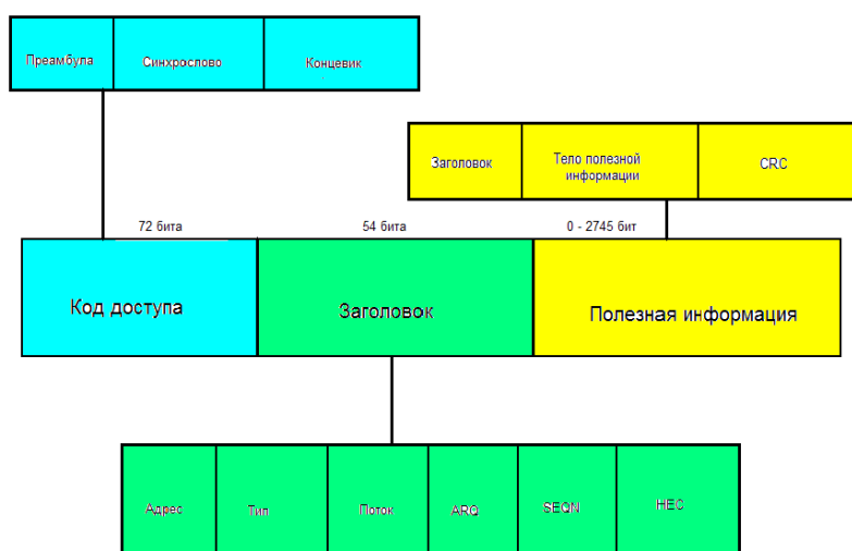
Рис. 7.89. Структура пакета
