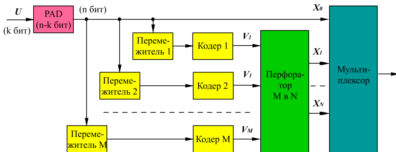
Рис. П1.74. Структурная схема турбо-кодера
