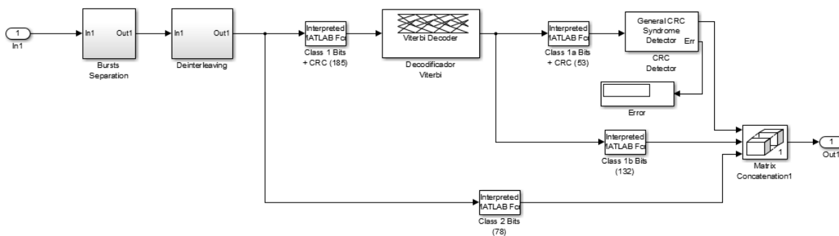
Рис. 7.8. Схема декодера
