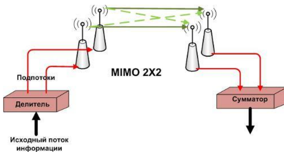
Рис. 7.123. MIMO 2x2
