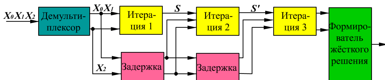
Рис. П1.76. Структурная схема трёх итерации турбо-декодера при двухкаскадном кодировании
