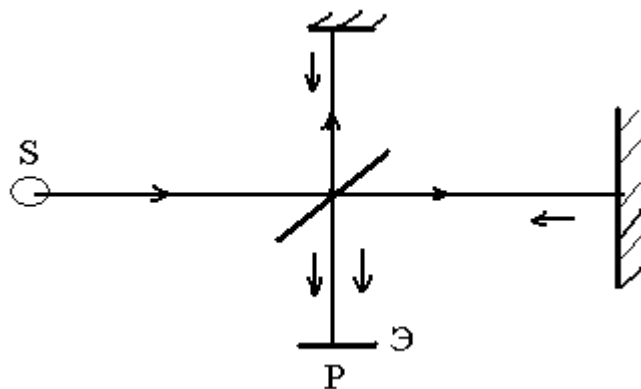
Рис. 2.2 — Схема интерферометра Майкельсона
