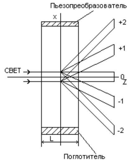
Рис. 10.6 — Дифракция Рамана-Ната
