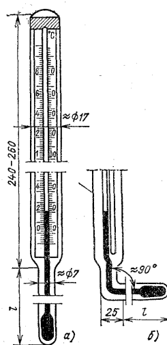
Рисунок 4. Технические стеклянные термометры
