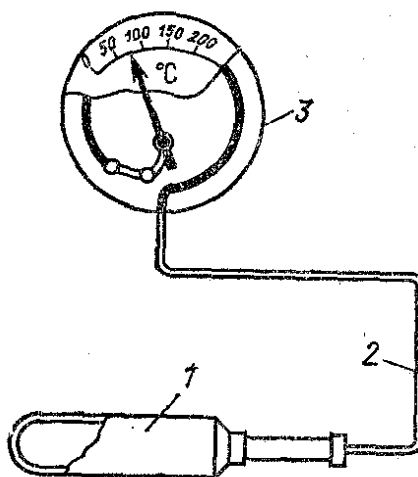
Рисунок 5. Манометрический термометр
