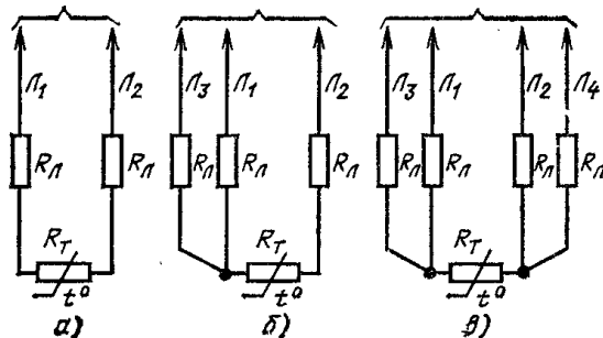
Рисунок 16. Схемы подсоединения термометров сопротивления
