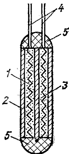
Рисунок 14. Чувствительный элемент платинового термометра сопротивления
