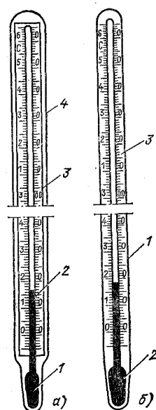
Рисунок 3. Лабораторные ртутные термометры:
