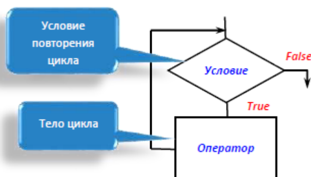
Рис. 6.4 – Цикл с предусловием while
