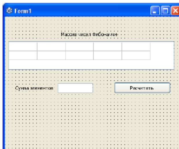
Рис. 6.6 – Интерфейс программы
