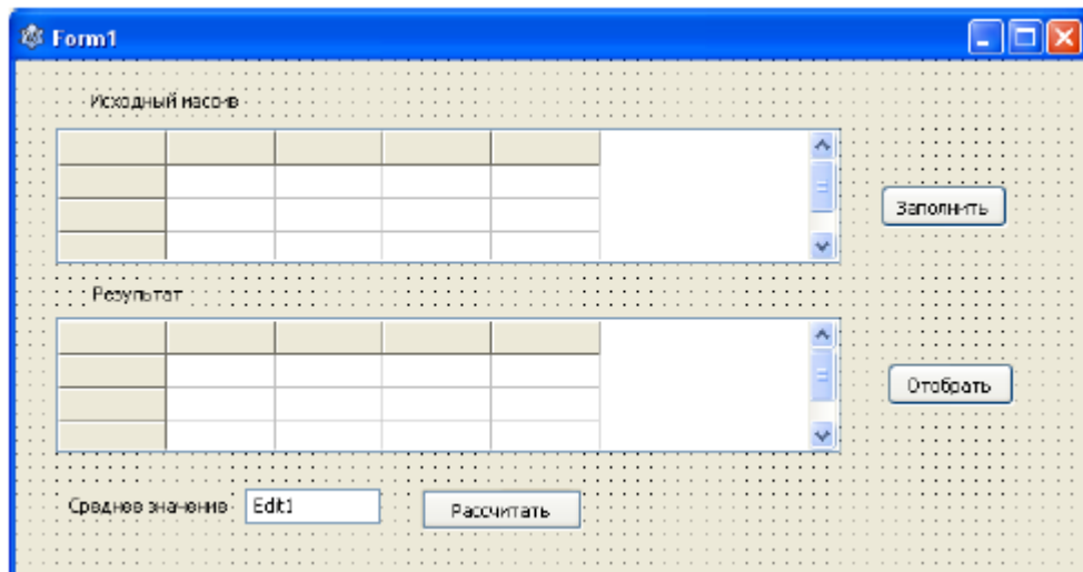
Рис. 7.3 - Интерфейс программы
