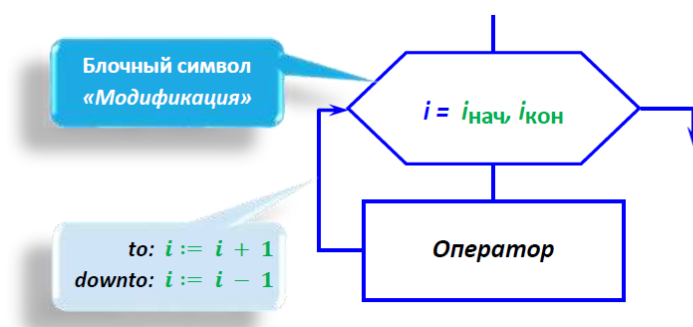
Рис. 5.6 – Изображение цикла for с помощью символа «Модификация»
