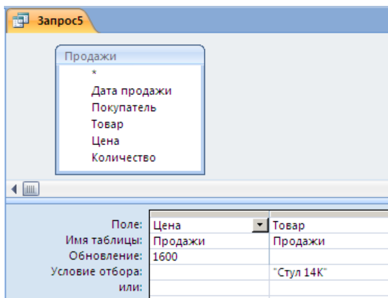
Рисунок 8.6 Запрос 5 на изменение данных
