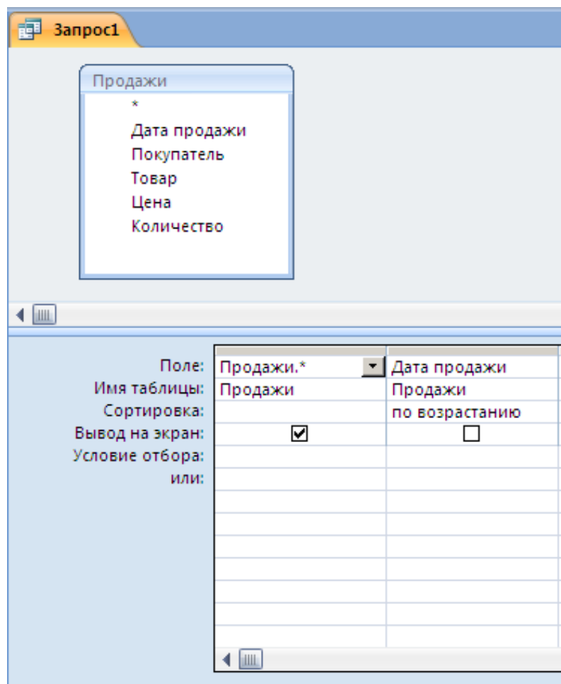
Рисунок 8.1 Запрос 1 в конструкторе MS Access
