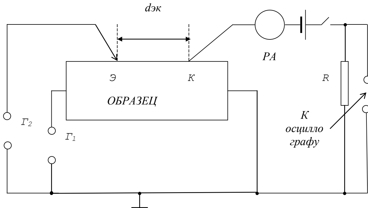
Рисунок 5.1. Схема установки для измерения подвижности неосновных неравновесных носителей заряда
