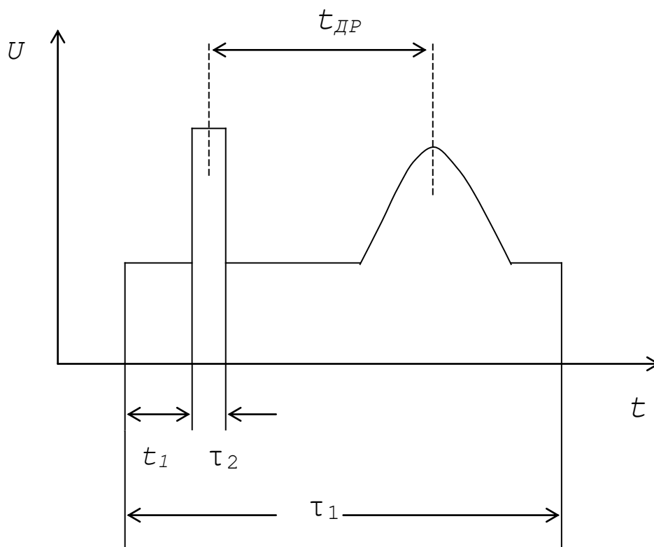
Рисунок 5.2. Осциллограмма импульсов
