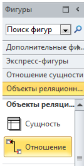
Рисунок 37 – Отношение (связь)
