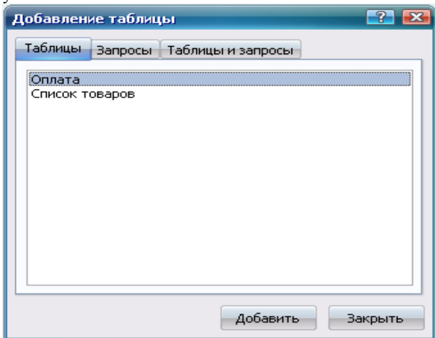
Рисунок 6 – Добавление таблицы
