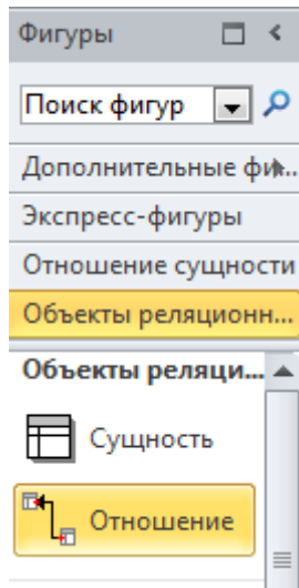
Рисунок 37 – Отношение (связь)
