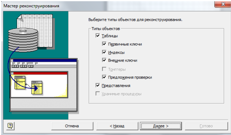
Рисунок 48 – Выбор объектов
