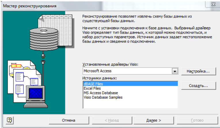
Рисунок 44 – Мастер реконструирования
