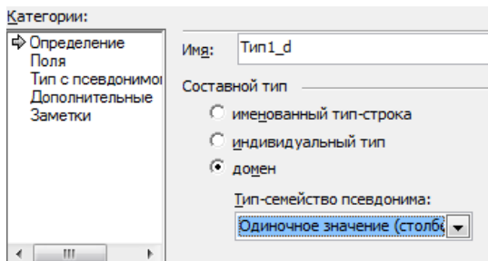
Рисунок 35 – Настройка домена
