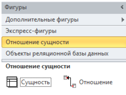
Рисунок 30 – Панель Фигуры
