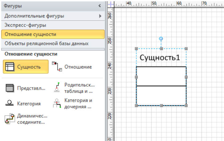
Рисунок 31 – Создание сущности
