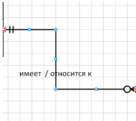
Рисунок 38 – Установленная связь
