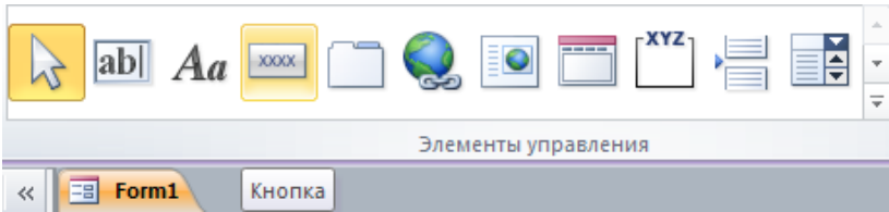
Рисунок 12 – Панель элементов
