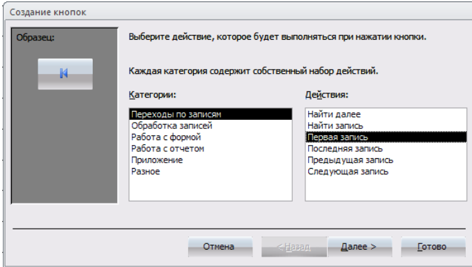
Рисунок 13 – Мастер кнопок
