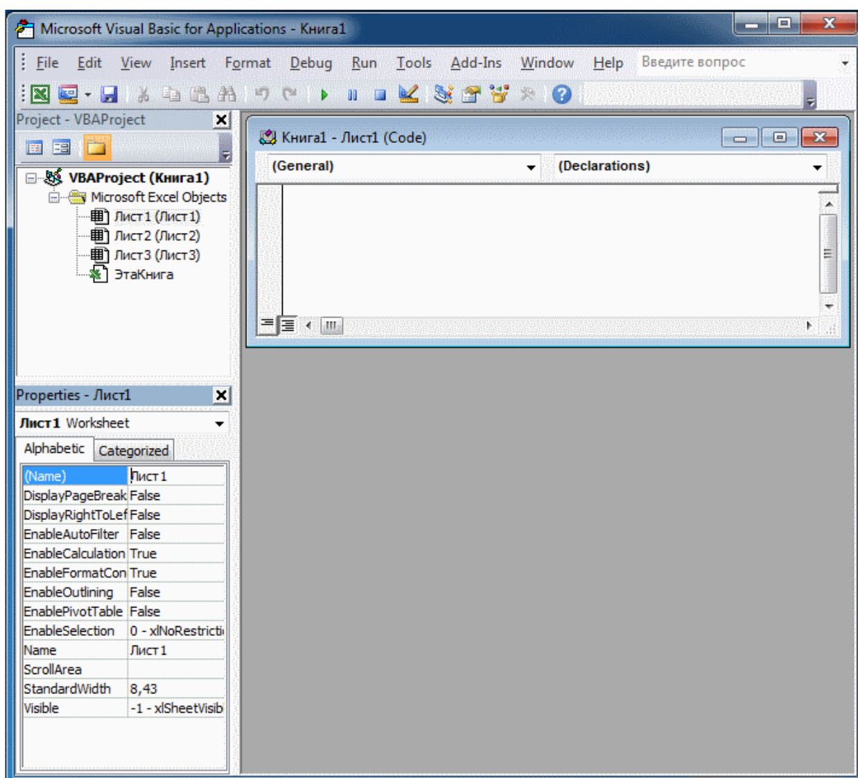
Рис. 5 Редактор VBA
