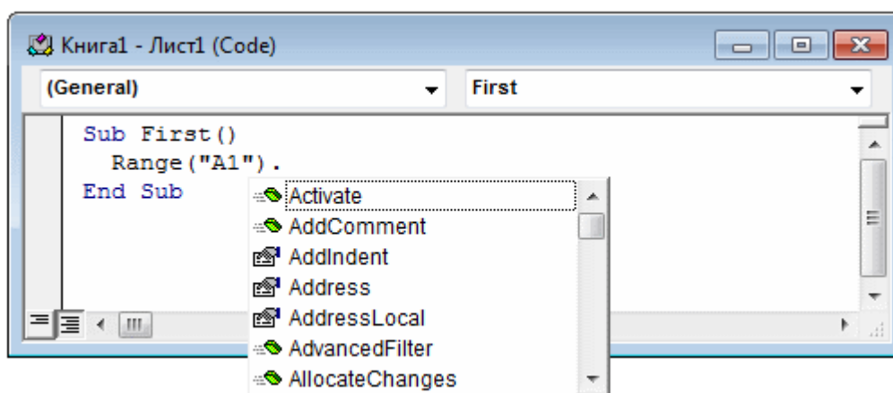
Рис. 9 Список компонентов
