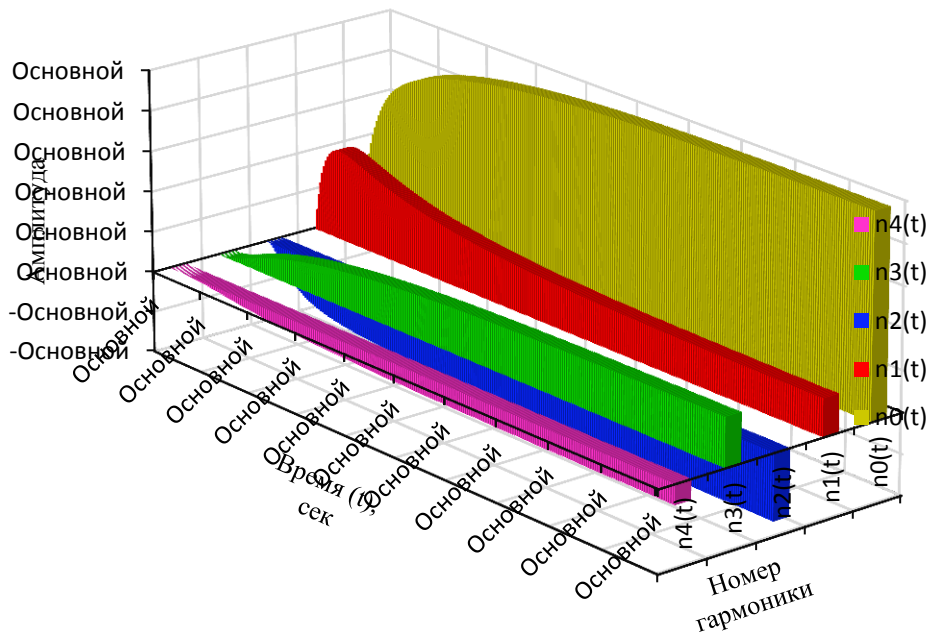
Рисунок 2.26 – Распределения гармоник показателя преломления n_0(t, j) , n_1(t, j) , n_2(t, j) , n_3(t, j) и n_4(t, j) при b = 0,1
