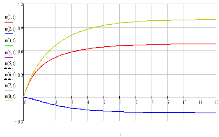
Рисунок 2.18 – Кинетика записи профилей гармоник показателя преломления n_0(t) , n_1(t) и n_2(t) при b = 2,1
