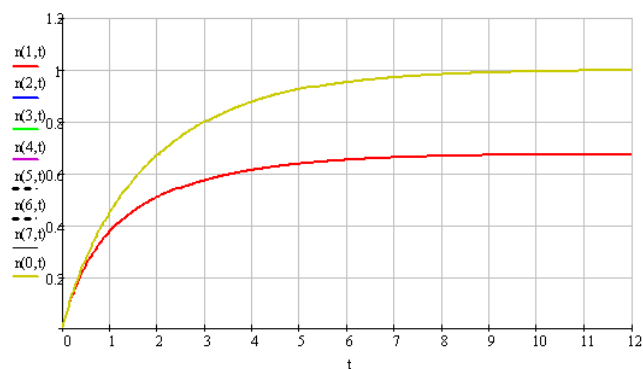
Рисунок 2.17 – Кинетика записи профилей гармоник показателя преломления n_0(t) и n_1(t) при b = 2,1
