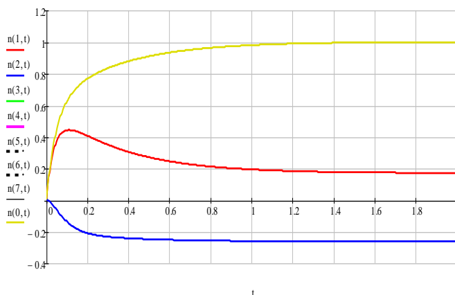
Рисунок 2.14 – Кинетика записи профилей гармоник показателя преломления n_0(t) , n_1(t) и n_2(t) при b = 0,1
