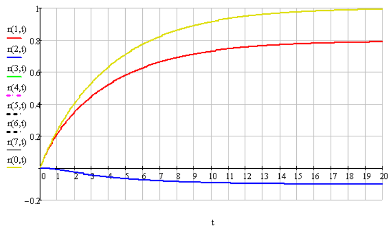
Рисунок 2.22 – Кинетика записи профилей гармоник показателя преломления n_0(t) , n_1(t) и n_2(t) при b = 5,1
