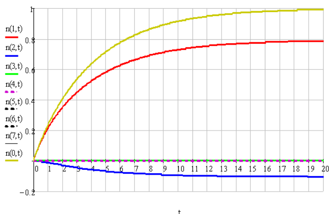
Рисунок 2.24 – Кинетика записи профилей гармоник показателя преломления n_0(t) , n_1(t) , n_2(t) , n_3(t) и n_4(t) при b = 5,1
