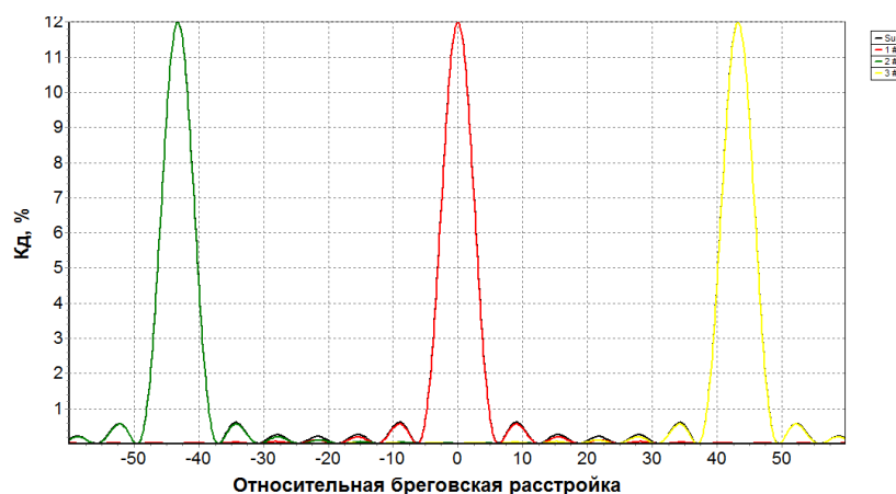
Рисунок 3.4 – Изменение дифракционной эффективности \eta_d решетки при отклонении от условий Брэгга с учетом автоматической оптимизации времени
