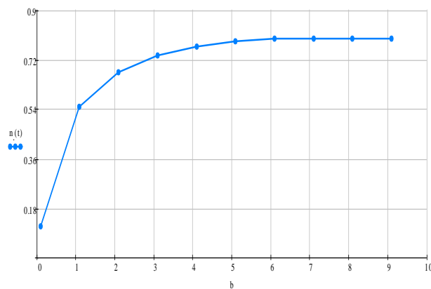
Рисунок 3.8 – Зависимость влияния параметра b = 0,1 \dots 9,1 на первую гармонику показателя преломления n_1(t = const)
