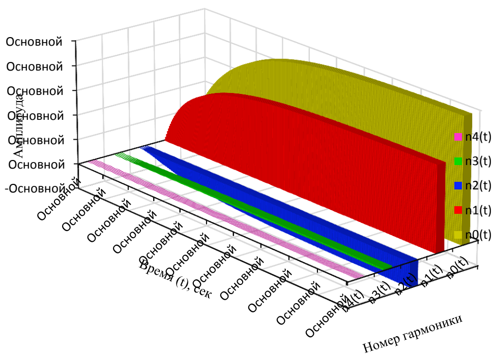
Рисунок 2.28 – Распределения гармоник показателя преломления n_0(t, j) , n_1(t, j) , n_2(t, j) , n_3(t, j) и n_4(t, j) при b = 2,1
