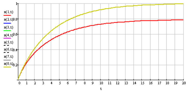
Рисунок 2.21 – Кинетика записи профилей гармоник показателя преломления n_0(t) и n_1(t) при b = 5 ,
