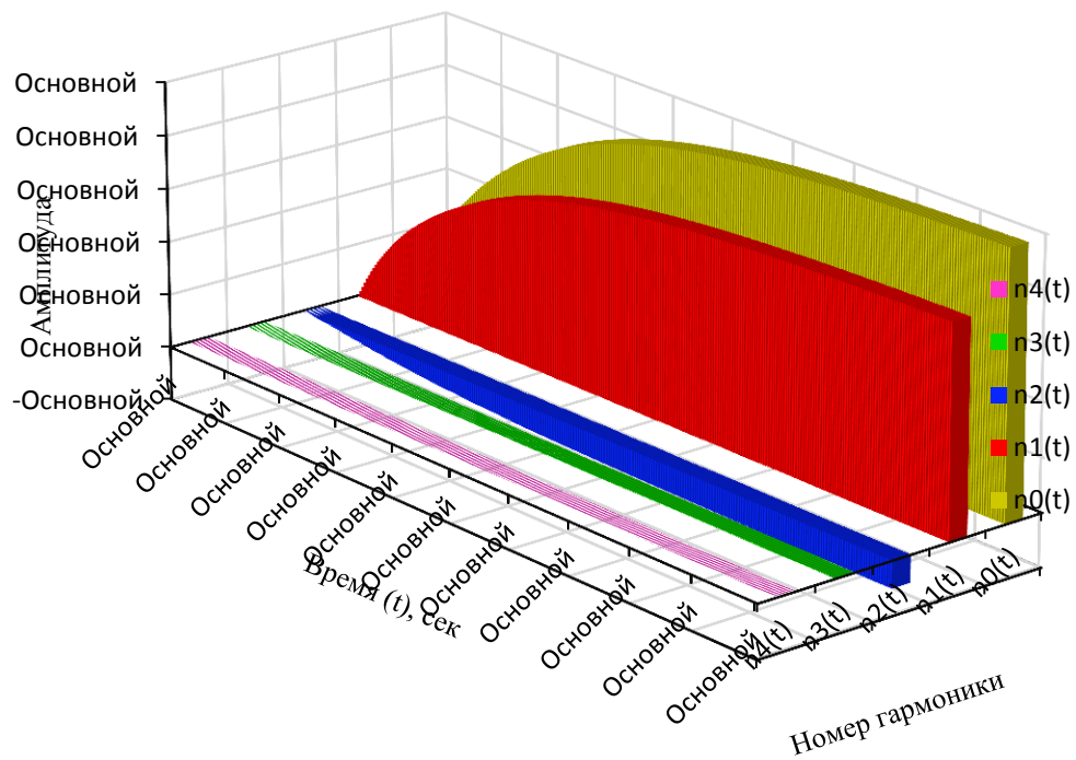
Рисунок 2.30 – Распределения гармоник показателя преломления n_0(t, j) ,
