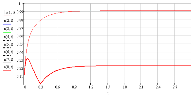
Рисунок 3.11 – Кинетика записи профилей гармоник показателя преломления n_0(t) и n_1(t) при \delta n_c = 3 и b = 0,1
