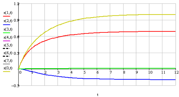
Рисунок 2.19 – Кинетика записи профилей гармоник показателя преломления n_0(t) , n_1(t) , n_2(t) и n_4(t) при b = 2,1
