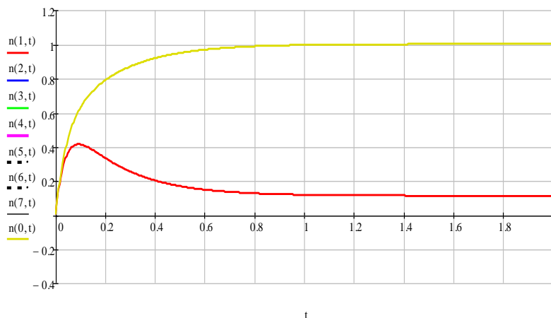
Рисунок 2.13 – Кинетика записи профилей гармоник показателя преломления n_0(t) и n_1(t) при b = 0,1
