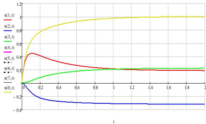
Рисунок 2.15 – Кинетика записи профилей гармоник показателя преломления n_0(t) , n_1(t) , n_2(t) и n_3(t) при b = 0,1
