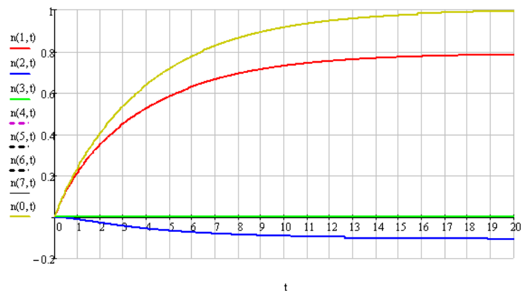
Рисунок 2.23 – Кинетика записи профилей гармоник показателя преломления n_0(t) , n_1(t) , n_2(t) и n_3(t) при b = 5,1
