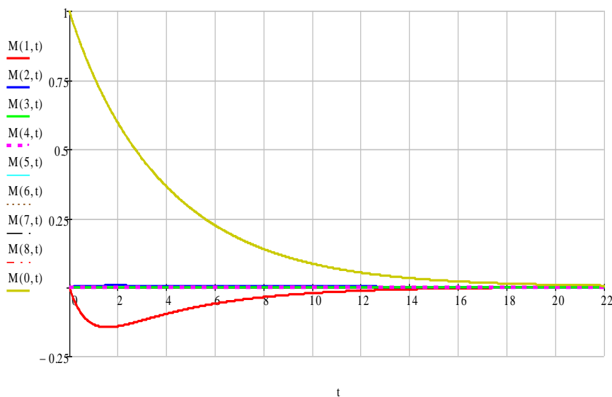
Рисунок 2.12 – Кинетика записи профилей гармоник концентрации мономера M_0(t) , M_1(t) , M_2(t) , M_3(t) и M_4(t) при b = 5,1
