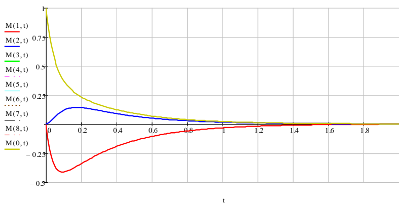
Рисунок 3.2 – Кинетика записи профилей гармоник концентрации мономера M_0(t) , M_1(t) и M_2(t) при b = 0,1
