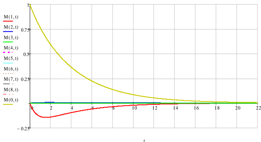
Рисунок 2.11 – Кинетика записи профилей гармоник концентрации мономера M_0(t) , M_1(t) , M_2(t) и M_3(t) при b = 5,1
