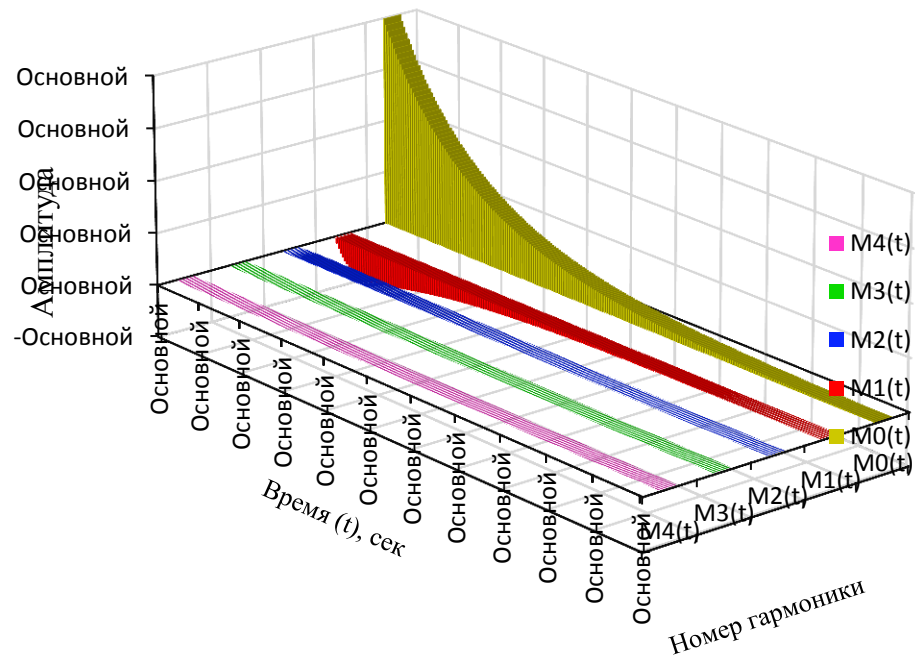
Рисунок 2.29 – Распределения гармоник концентрации мономера M_0(t, j) , M_1(t, j) , M_2(t, j) , M_3(t, j) и M_4(t, j) при b = 5,1
