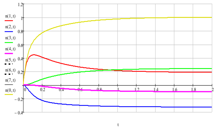
Рисунок 2.16 – Кинетика записи профилей гармоник показателя преломления n_0(t) , n_1(t) , n_2(t) , n_3(t) и n_4(t) при b = 0,1
