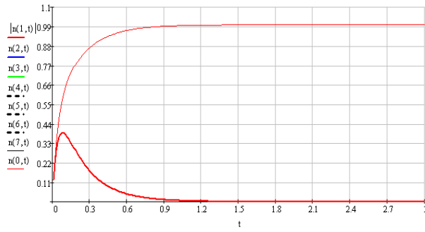
Рисунок 3.10 – Кинетика записи профилей гармоник показателя преломления n_0(t) и n_1(t) при \delta n_c = 1 и b = 0,1
