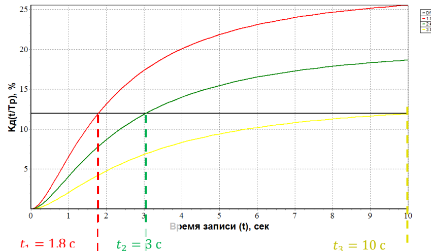
Рисунок 3.5 – Зависимость дифракционной эффективности каждой решетки от времени записи при последовательном угловом мультиплексировании с учетом автоматической оптимизации t
