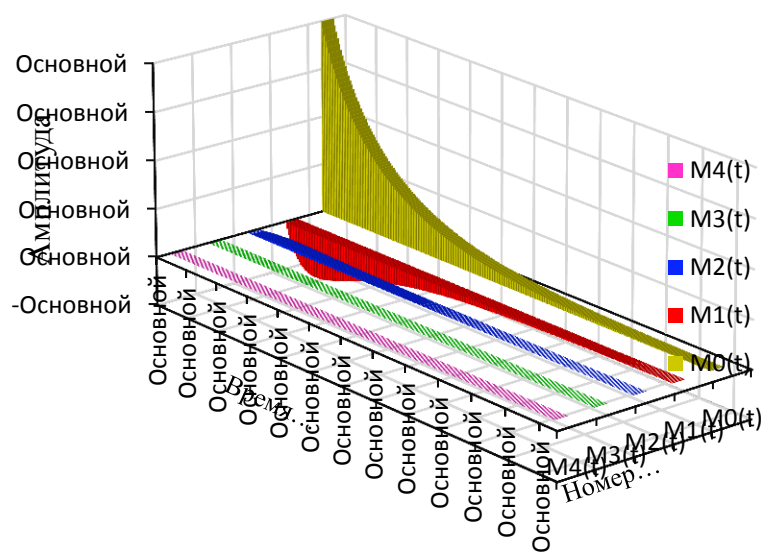
Рисунок 2.27 – Распределения гармоник концентрации мономера M_0(t, j) , M_1(t, j) , M_2(t, j) , M_3(t, j) и M_4(t, j) при b = 2,1
