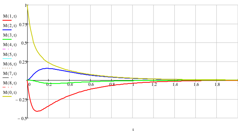
Рисунок 3.3 – Кинетика записи профилей гармоник концентрации мономера M_0(t) , M_1(t) , M_2(t) и M_3(t) при b = 0,1
