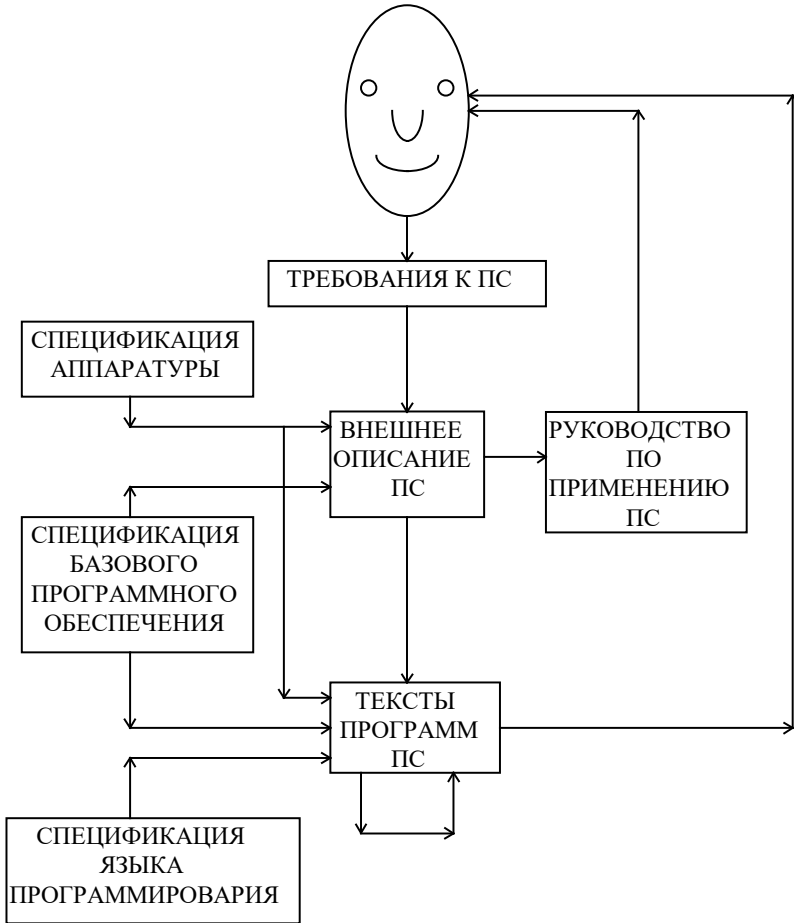
Рис. 2.1. Грубая схема разработки и применения ПС
