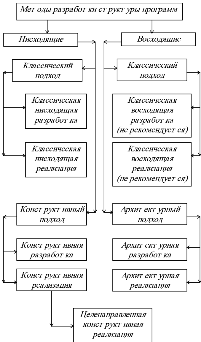
Рис. 6.3. Классификация методов разработки структуры программ.
