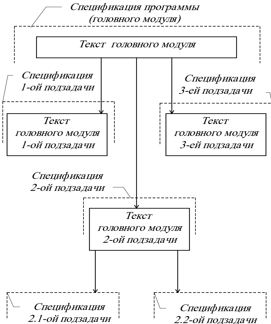
Рис. 6.2. Второй шаг формирования модульной структуры программы при конструктивном подходе.
