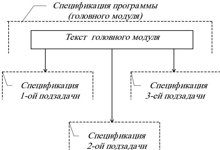
Рис. 6.1. Первый шаг формирования модульной структуры программы при конструктивном подходе
