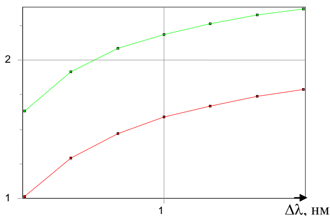
Рисунок 3.6.1 - Зависимость G_{max}(\Delta\lambda)
