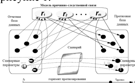
Рисунок 1. Схема прогнозирования в «АИС-Регион»
