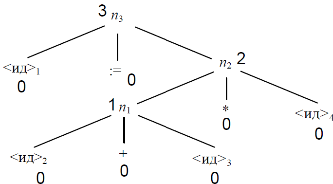
Рисунок 3 — Дерево разбора с уровнями
