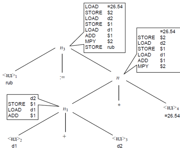
Рисунок 4 — Дерево разбора с кодами
