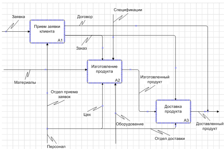
Рисунок 1.8. Диаграмма декомпозиции 1-го уровня
