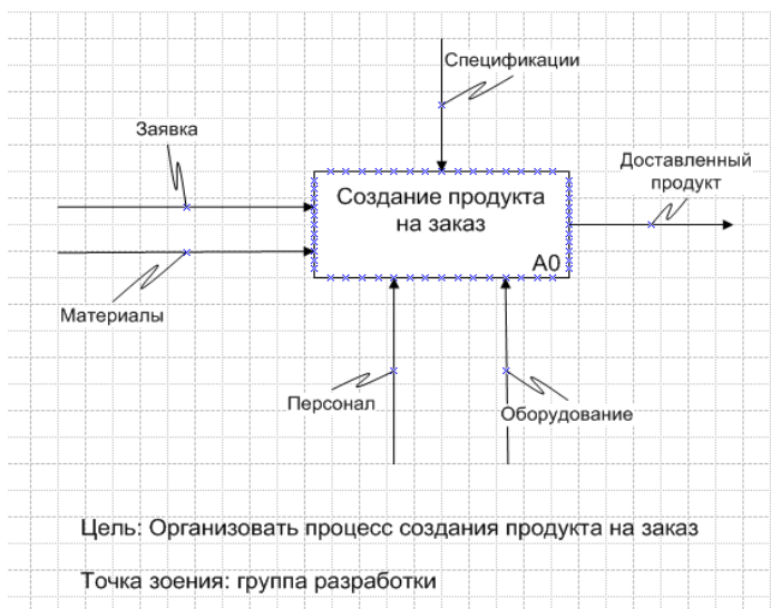
Рисунок 1.7. Пример контекстной диаграммы
