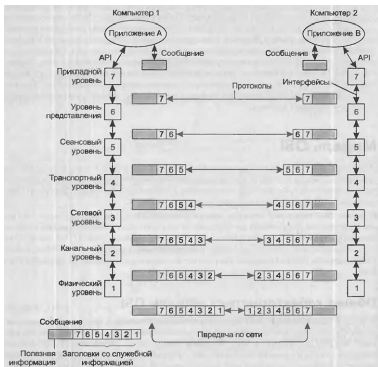
Рисунок 4.1 — Модель взаимодействия открытых систем ISO / OSI [1].
