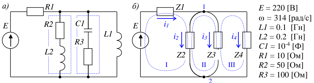
Рис. 65 – Расчет цепи переменного тока
