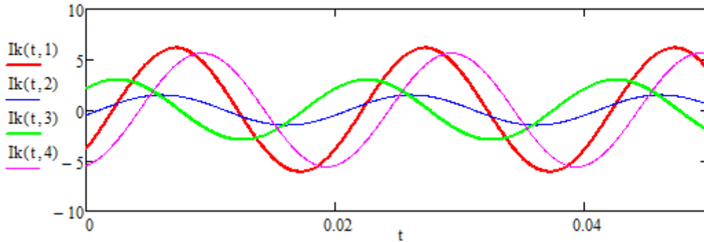
Рис. 67 – Токи в цепи переменного тока
