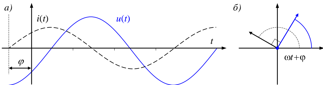
Рис. 64 – Ток и напряжение на конденсаторе
