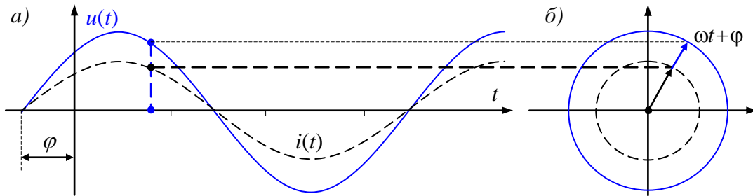
Рис. 62 – Ток и напряжение на резисторе
