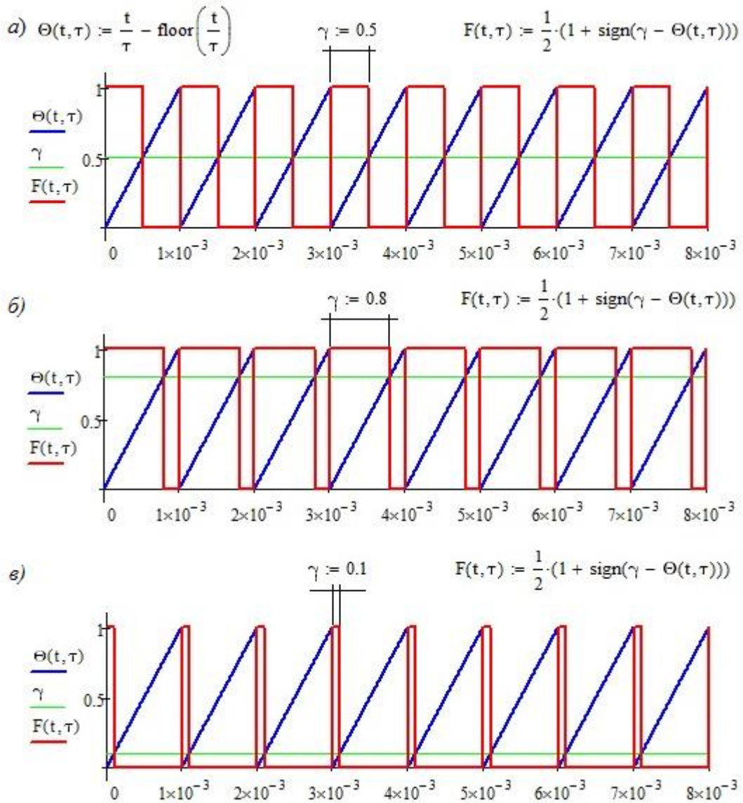
Рис. 29 – Широтно-импульсная модуляция
