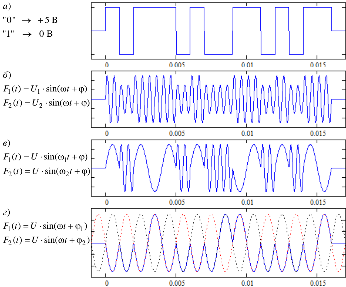
Рис. 32 – Виды аналоговой модуляции
