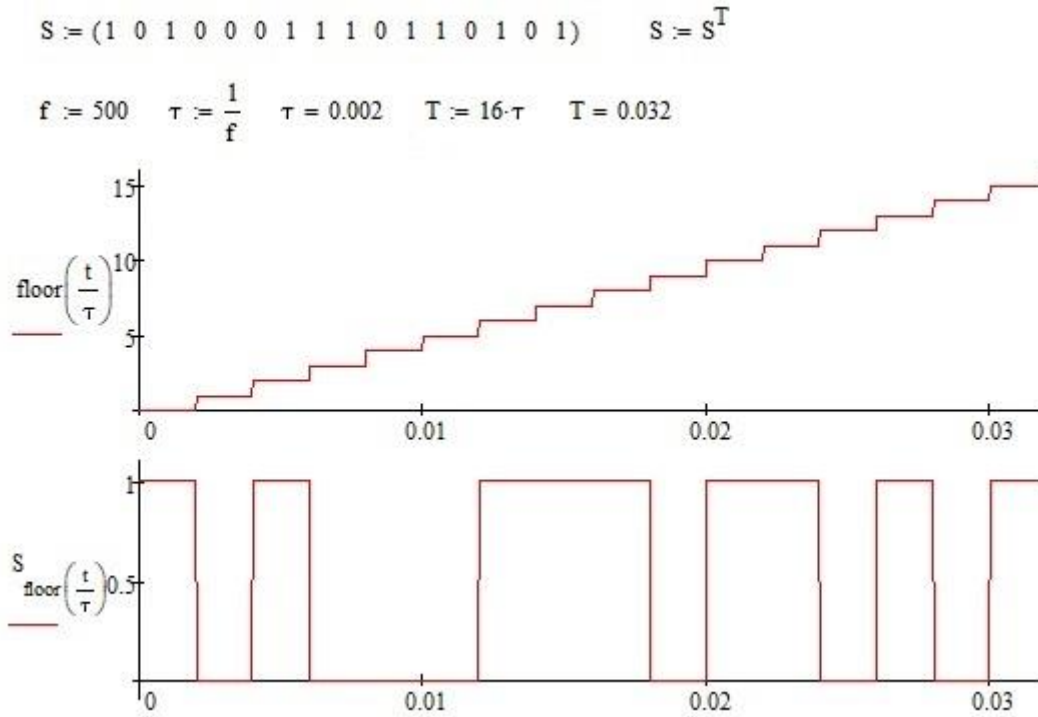
Рис. 33 – Импульсная последовательность
