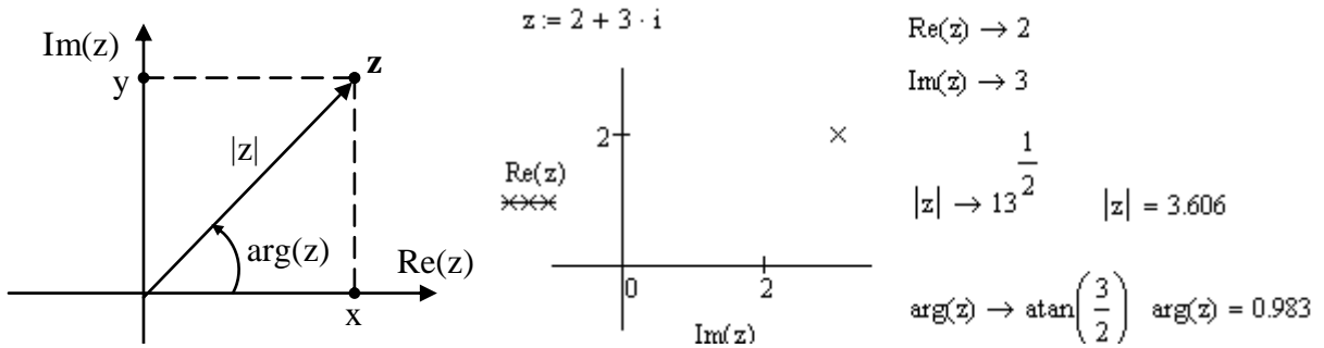
Рис. 54 – Представление комплексного числа в MathCAD
