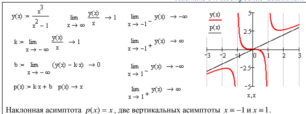
Листинг 14. Построение асимптот
