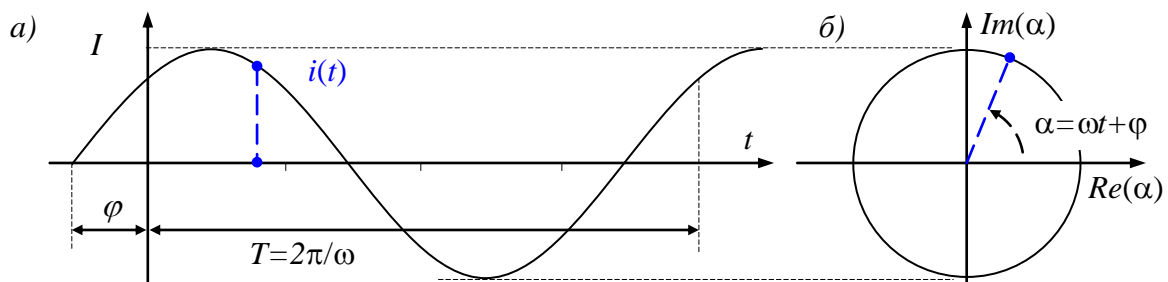
Рис. 61 – Представление (а) гармонического сигнала в виде (б) комплексной величины
