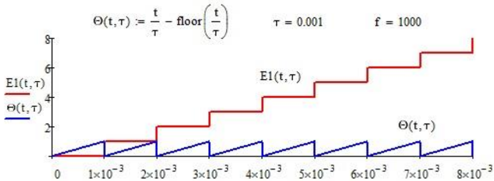
Рис. 27 – График линейно-нарастающей функции \Theta(t, \tau)
