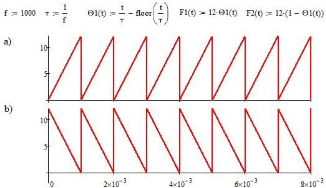
Рис. 24 – График (а) линейно-растущей и (б) линейно-спадающей периодических функций
