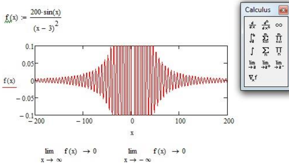
Рис. 11 - Вычисление пределов функции на +\infty и на -\infty
