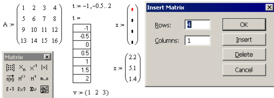
Рис. 40 – Матрицы и вектора в MathCAD. Диалоговое окно ввода матрицы
