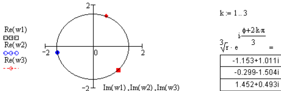
Рис. 58 – Пример многозначной функции \sqrt[3]{2 + 3i}
