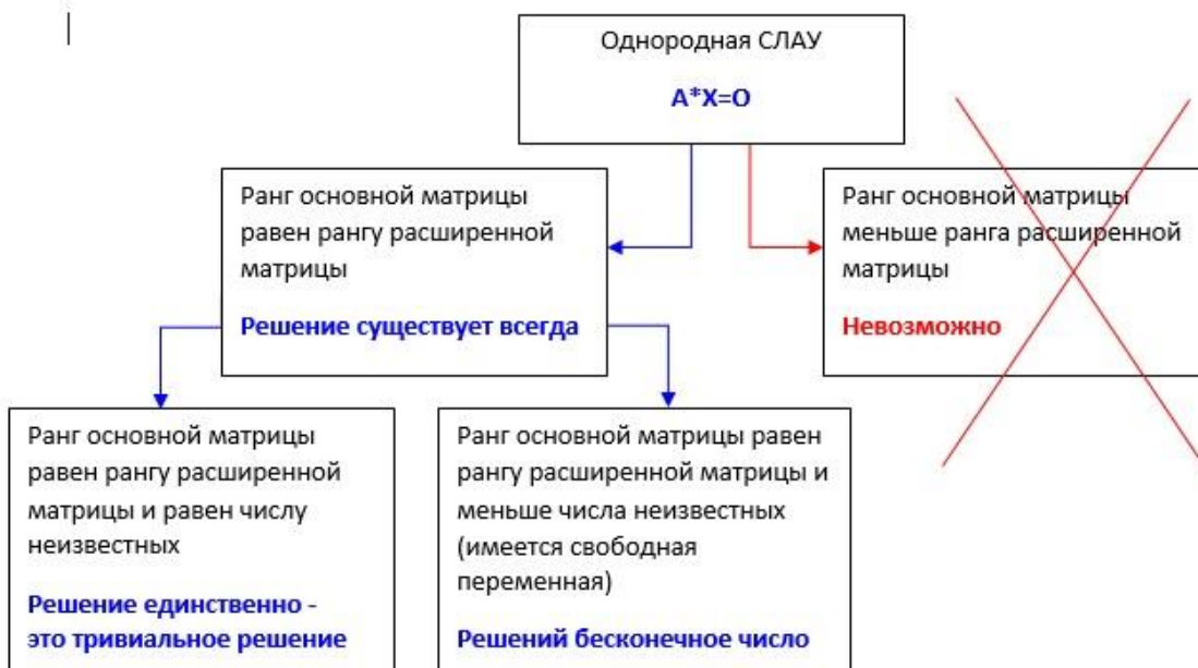
Рис. 47 – Существование и единственность решений однородной СЛАУ
