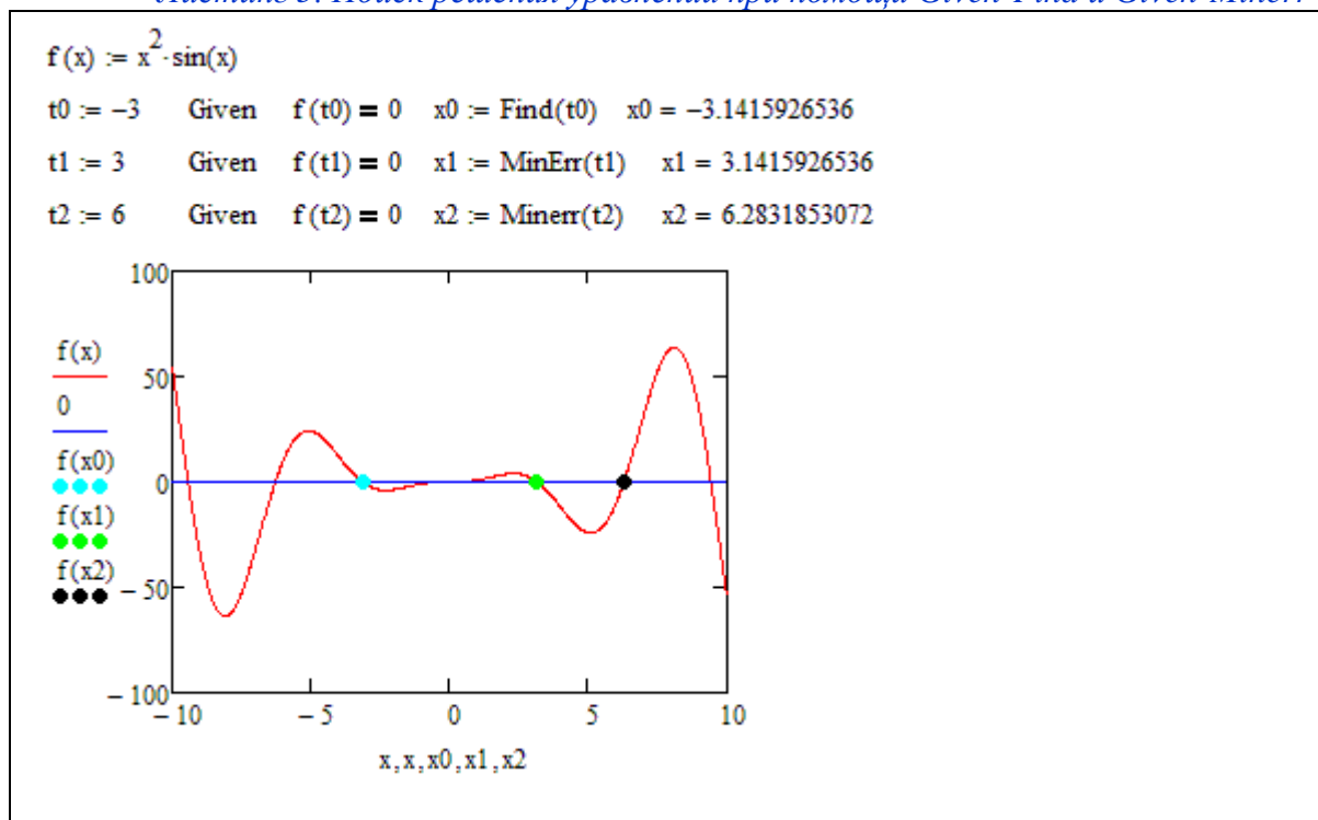
Листинг 5. Поиск решения уравнений при помощи Given-Find и Given-Minerr
