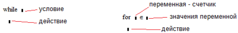
Рис. 20 – Структура операторов while и for
