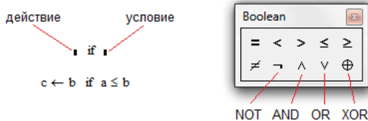
Рис. 19 – Структура оператора if . Блок ввода логических команд
