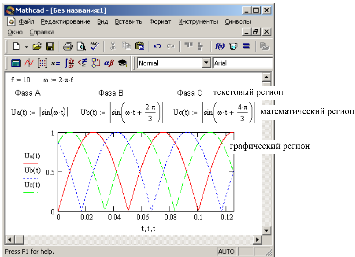
Рис. 3 – Окно интерфейса MathCAD с загруженным документом
