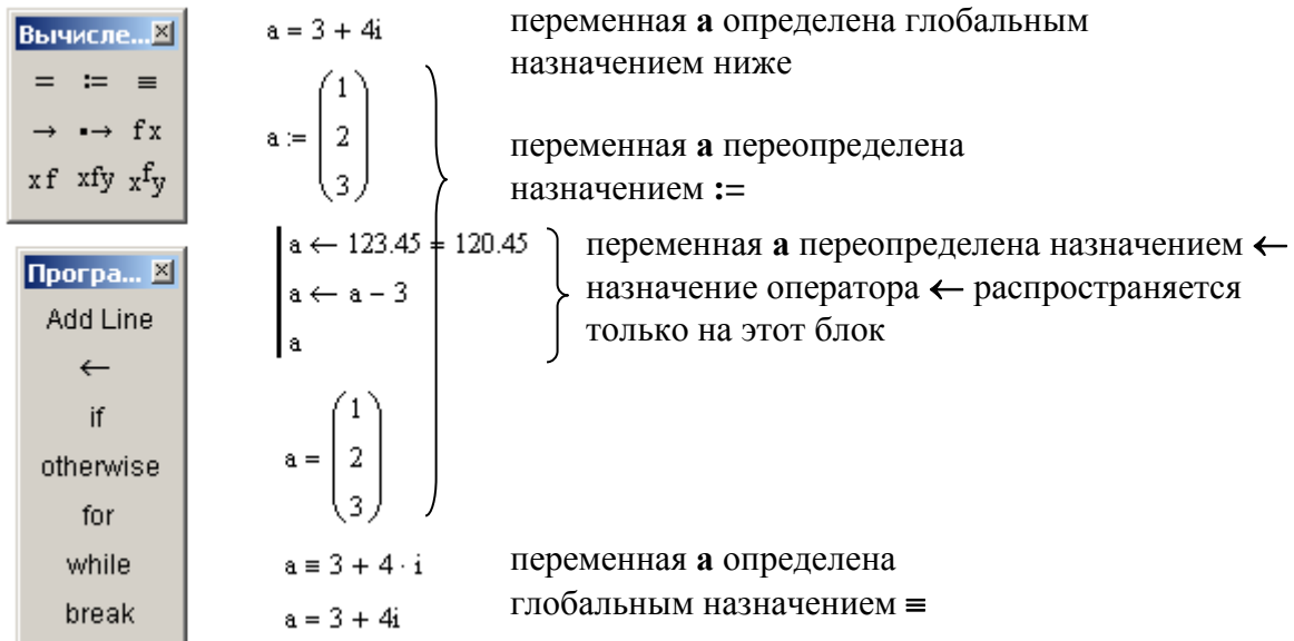
Рис. 6 – Области действия (видимости) операторов назначения
