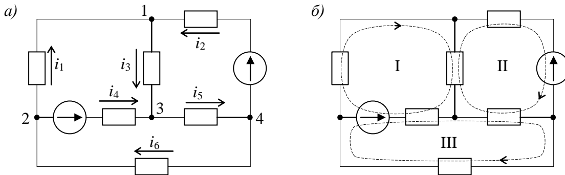
Рис. 51 – а) условные направления токов в ветвях схемы; б) направления обхода контуров
