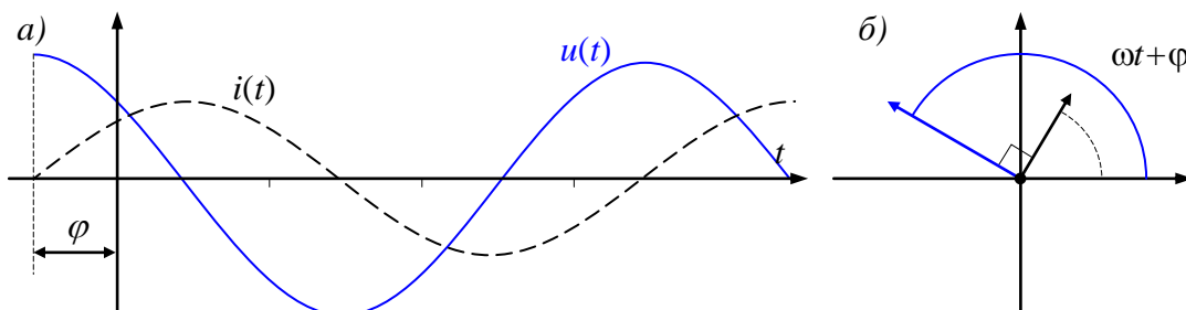
Рис. 63 – Ток и напряжение в катушке индуктивности
