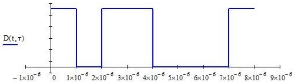
Рис. 31 – График двоичной последовательности S с тактовым периодом \tau = 10^{-6} [с]
