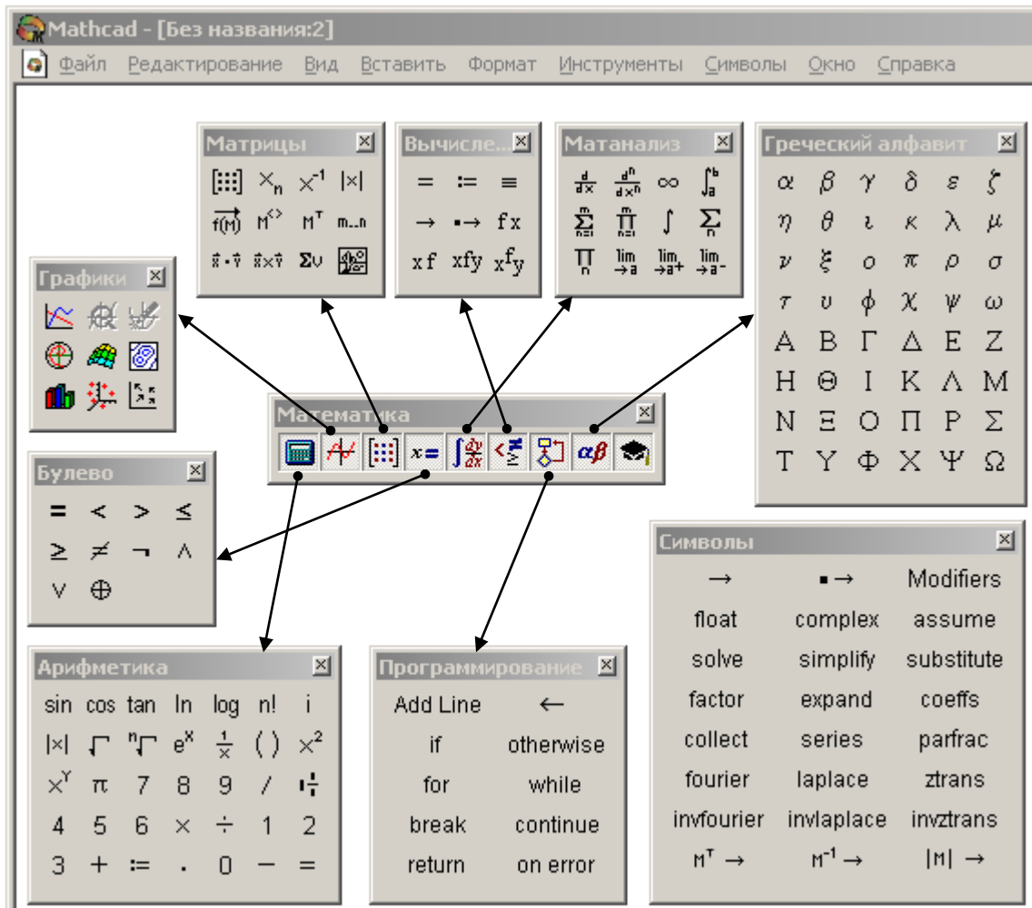
Рис. 4 – Панели инструментов и линейка их вызова
