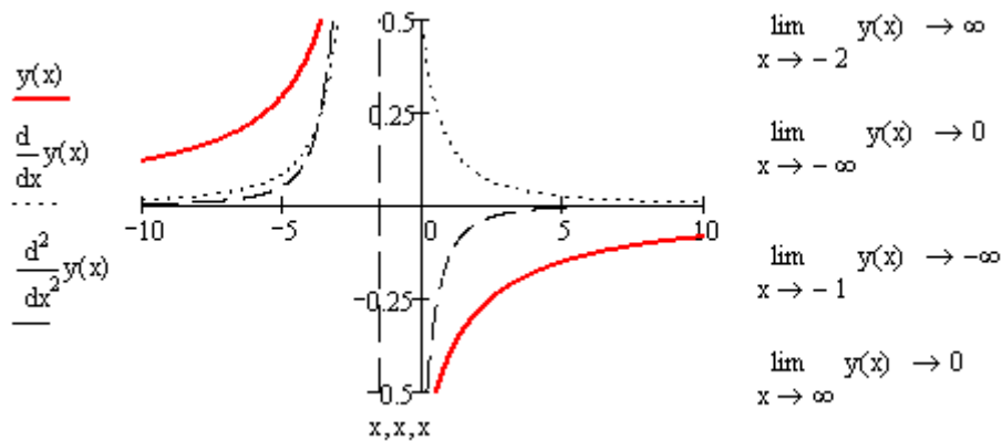
Рис. 14 – Исследование экстремумов и перегибов (2)
