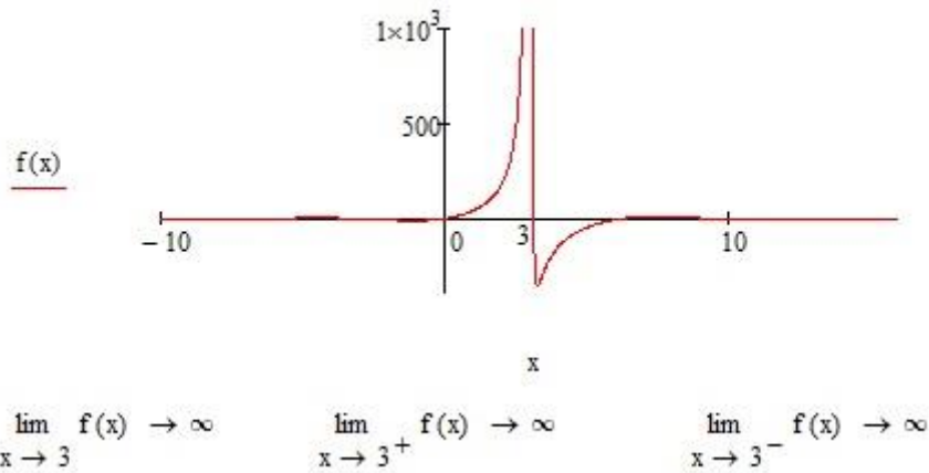
Рис. 12 - Вычисление пределов функции справа и слева в точке
