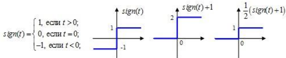
Рис. 28 – Сигнум функция и её модификации
