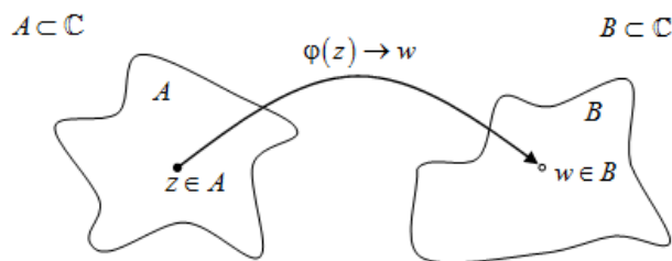
Рис. 57 – Представление комплексных функций
