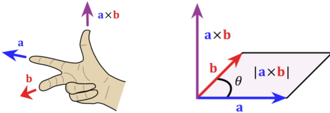
Рис. 43 – Результат векторного произведения направлен так, чтобы образовывать правую тройку векторов
