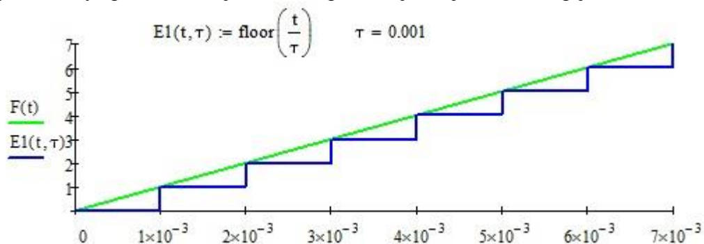
Рис. 26 – График ступенчатой функции с интервалами \tau
