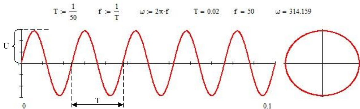
Рис. 22 – Основные параметры гармонической функции
