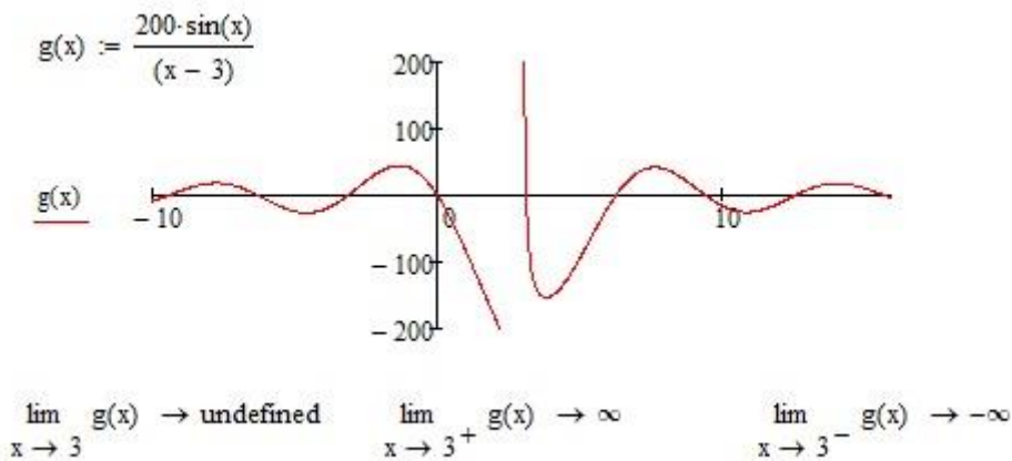
Рис. 13 - Вычисление пределов функции справа и слева в точке
