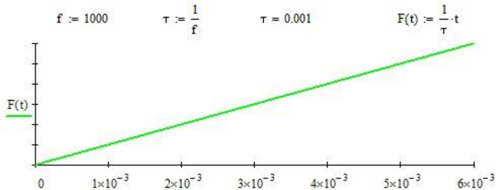
Рис. 25 – График линейной функции с наклоном 1/\tau
