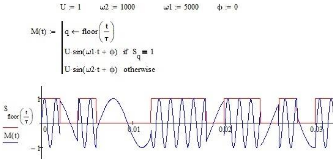
Рис. 35 – Частотная модуляция
