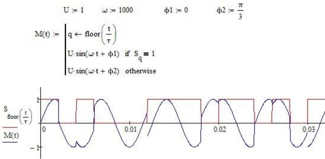
Рис. 36 – Фазовая модуляция
