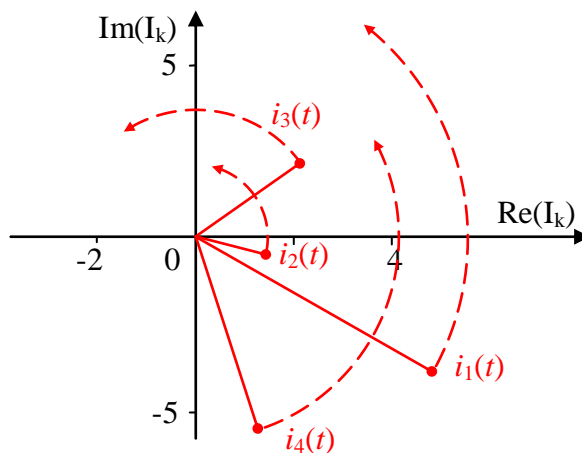
Рис. 66 – Токи в цепи переменного тока представленные в виде вращающихся комплексных векторов
