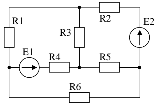
Рис. 50 – Задача на баланс мощностей в цепи постоянного тока
