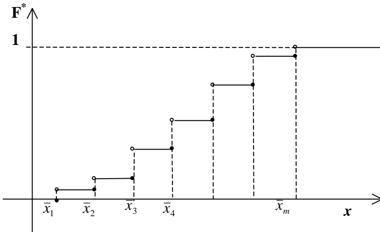
Рис 3. Эмпирическая функция распределения.
