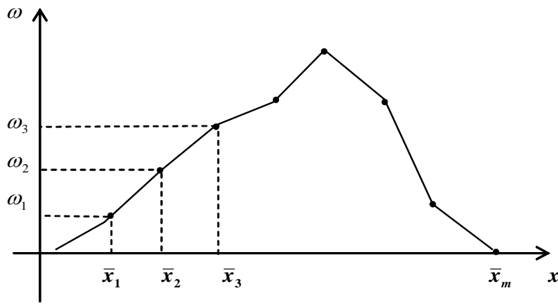
Рис. 1.1. Полигон частот
