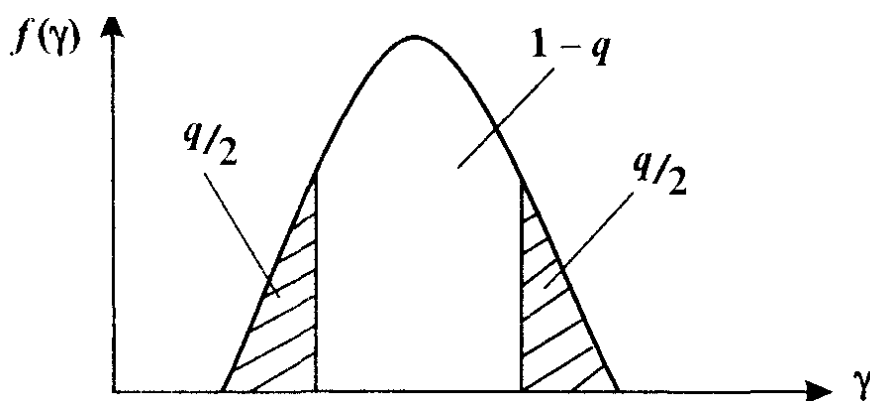
Рис. 5.1 График плотности распределения критической статистики \gamma .
