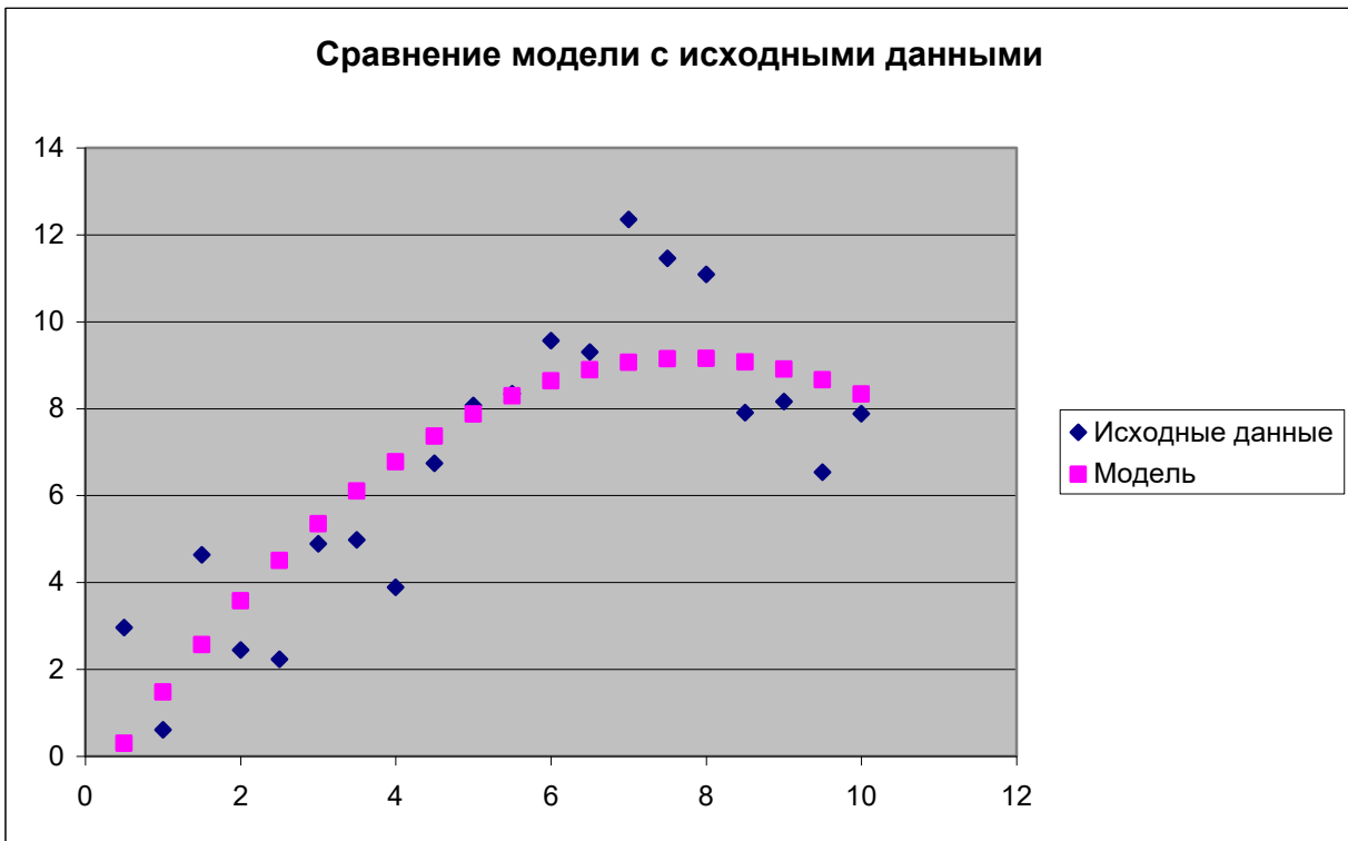
Рис. 8.2. Сравнение модели y = \beta_0 + \beta_1 x + \beta_2 x^2 с исходными данными
