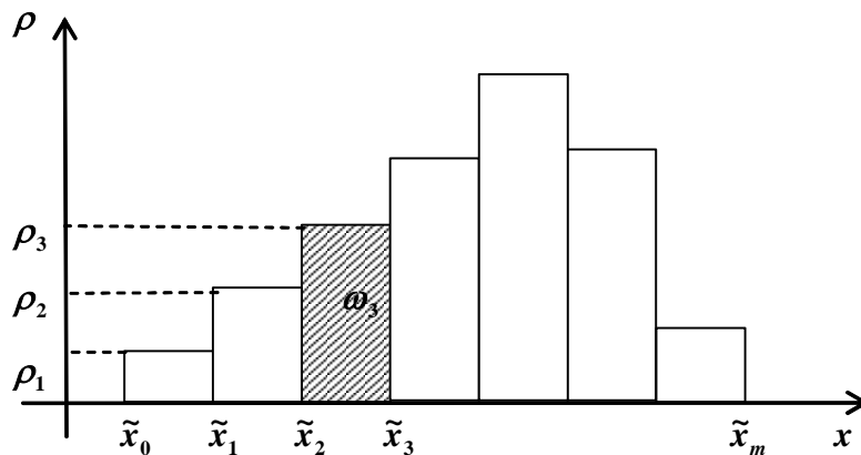
Рис 2. Гистограмма частот.
