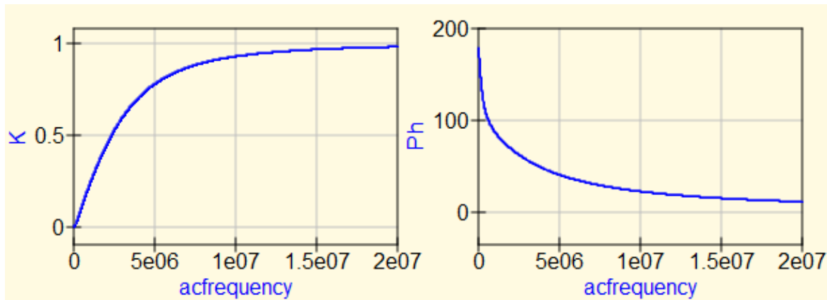
Рис. Б.13 – АЧХ и ФЧХ передаточной функции
