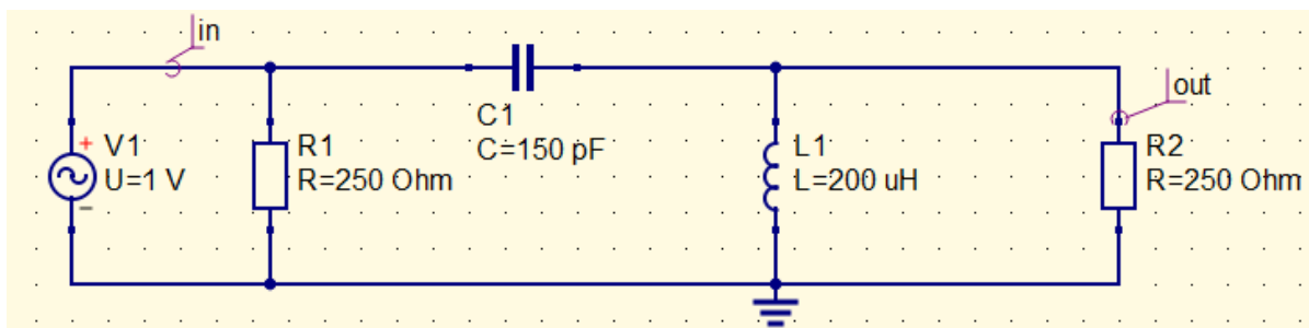
Рис. Б.6 – Схема для моделирования в QUCS
