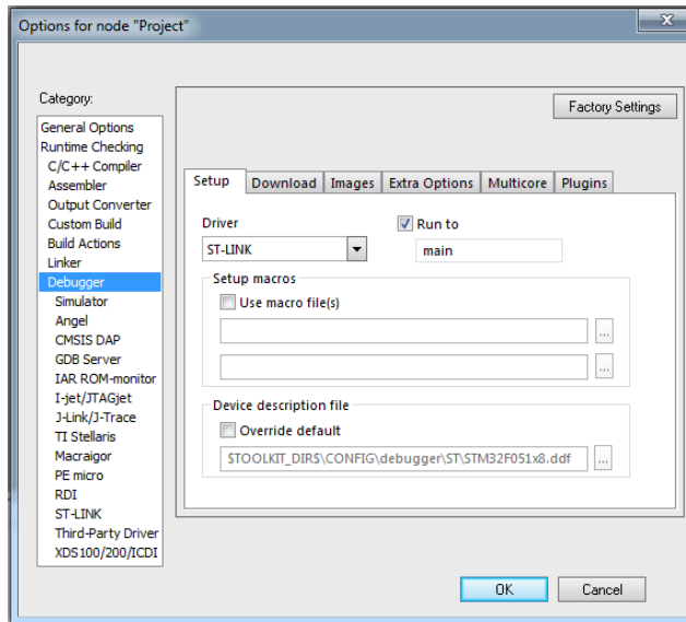
Рисунок 3.8 – Установка типа отладчика
