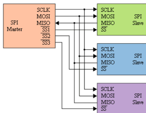
Рисунок 4.5 – Соединение с несколькими Ведомыми
