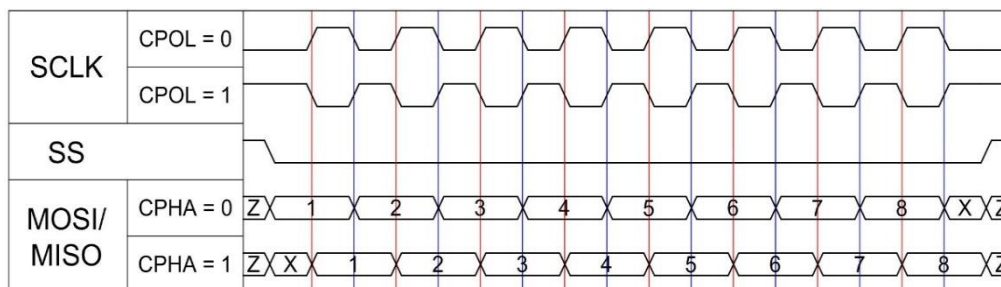
Рисунок 4.6 – Режимы SPI
