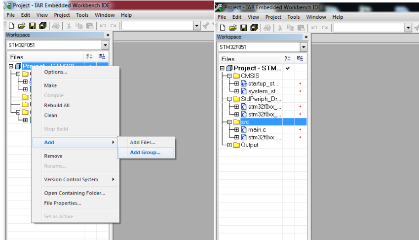
Рисунок 3.4 – Результат.
