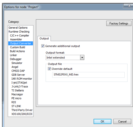
Рисунок 3.7 – Вкладка «OutputConverter»
