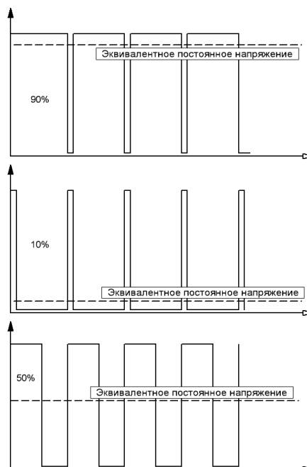
Рисунок 4.3 – ШИМ с разной длиной импульса
