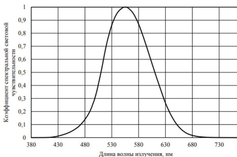
Рисунок 1 – Фотопическая функция
