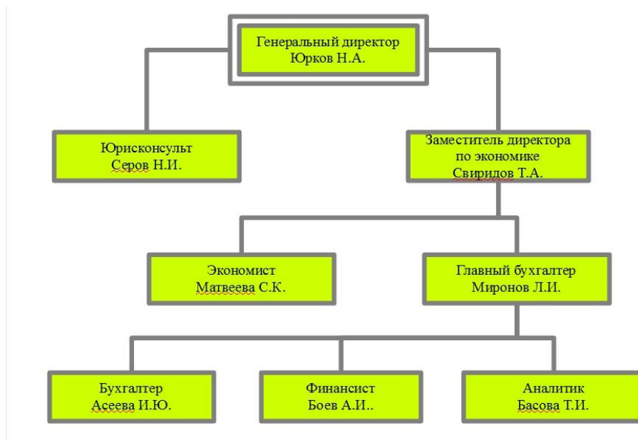
Рисунок 9.7 – Соединение фигур
