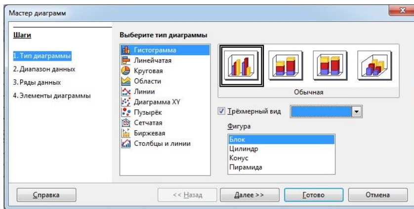
Рисунок 4.3 – Мастер диаграмм
