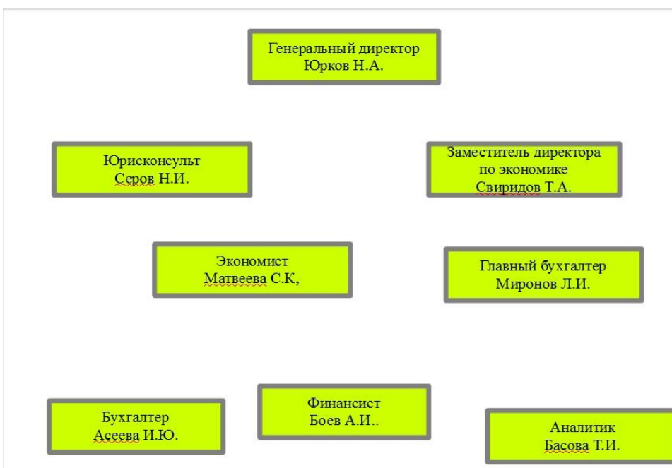
Рисунок 9.4 – Изменение текста
