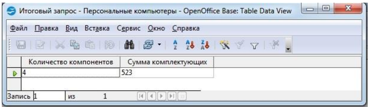
Рисунок 8.6 – Итоговый запрос
