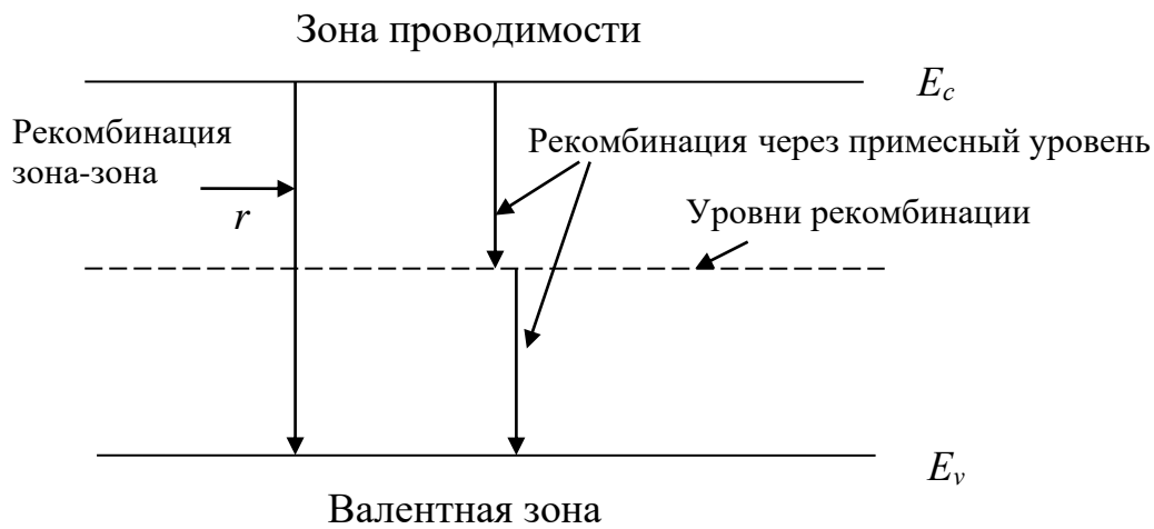
Рисунок 2.2 – Возможные механизмы рекомбинации носителей заряда
