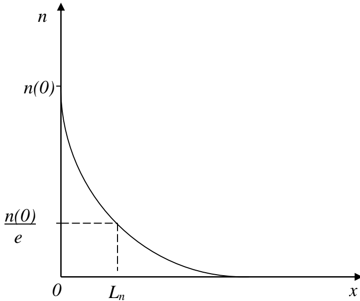
Рисунок 4.2 Зависимость концентрации неравновесных носителей заряда от расстояния.
