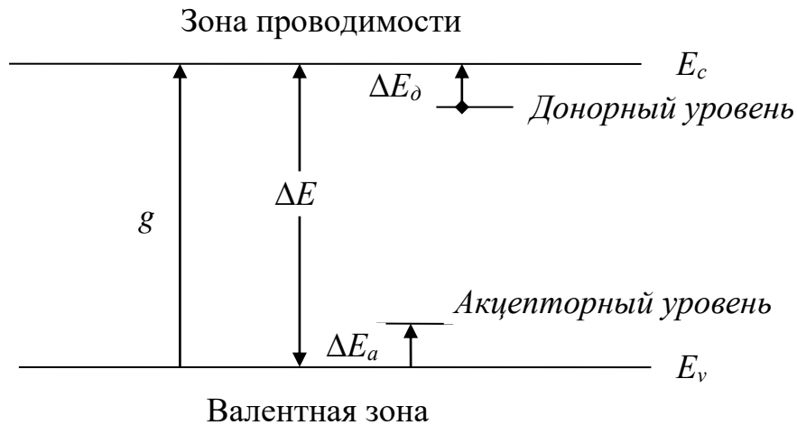
Рисунок 2.1 – Возможные механизмы генерации носителей заряда
