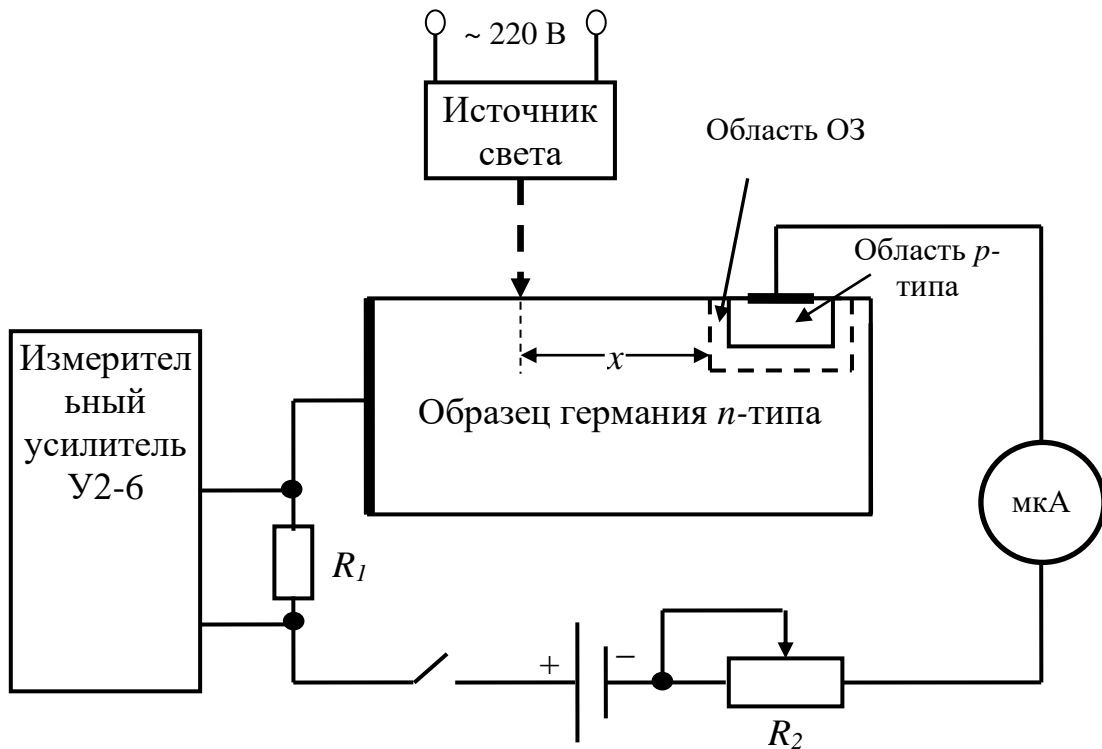
Рисунок 5.1 – Схема установки для измерения диффузионной длины неосновных носителей заряда
