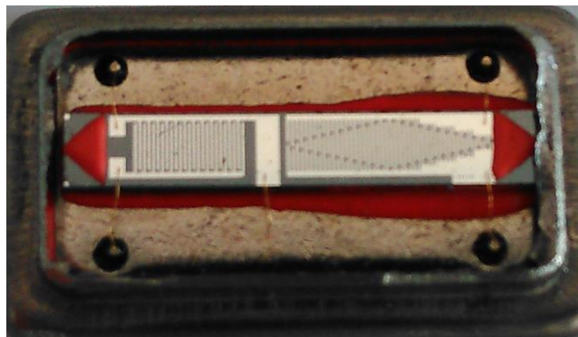
Рисунок 6 – Структура полосового фильтра К04ФЕ003
