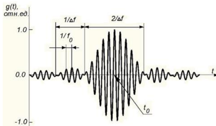
Рисунок 3 – Пять лепестков импульсной характеристики фильтра на ПАВ
