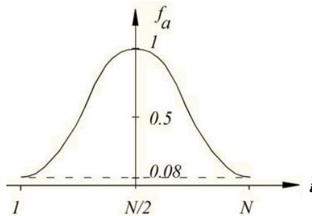
Рисунок 5 – Функция аподизации Хемминга
