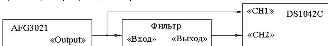
Рисунок 8 – Структурная схема измерений частотной и импульсной характеристик фильтра
