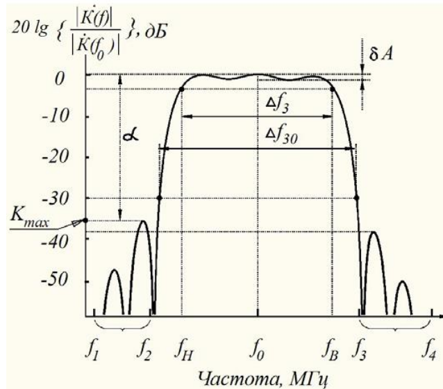
Рисунок 4 – К определению основных параметров фильтра
