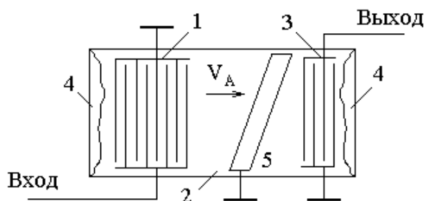
Рисунок 1 – Базовая конструкция фильтра на ПАВ
